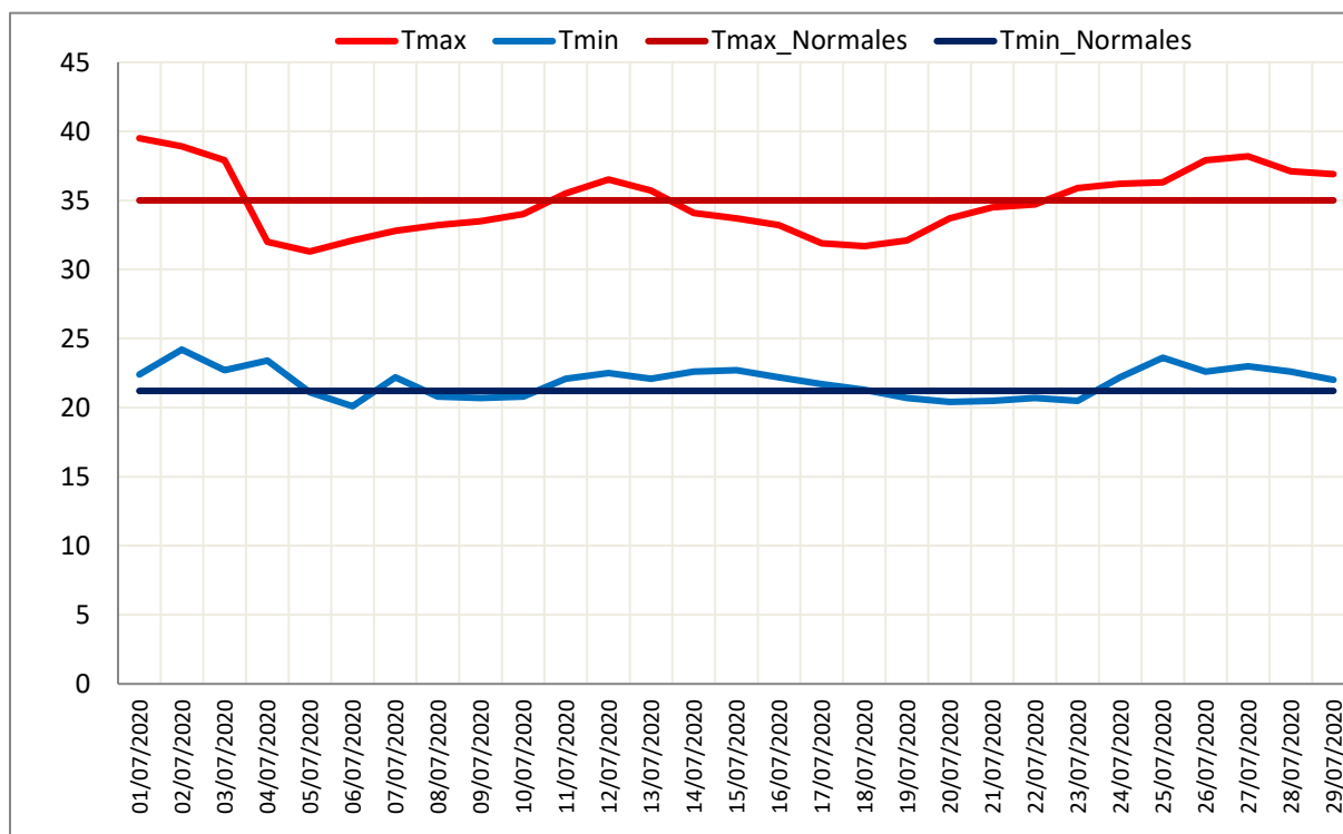
Evolutions des températures maximales et minimales quotidiennes en Tunisie par rapport à la normale du mois de Juillet
