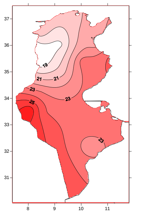
Température minimale en (°C)
