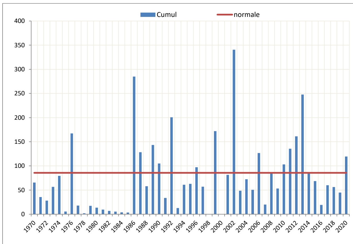
Cumul mensuel des précipitations sur les 50 dernières années sur la Tunisie: mois de Juillet
