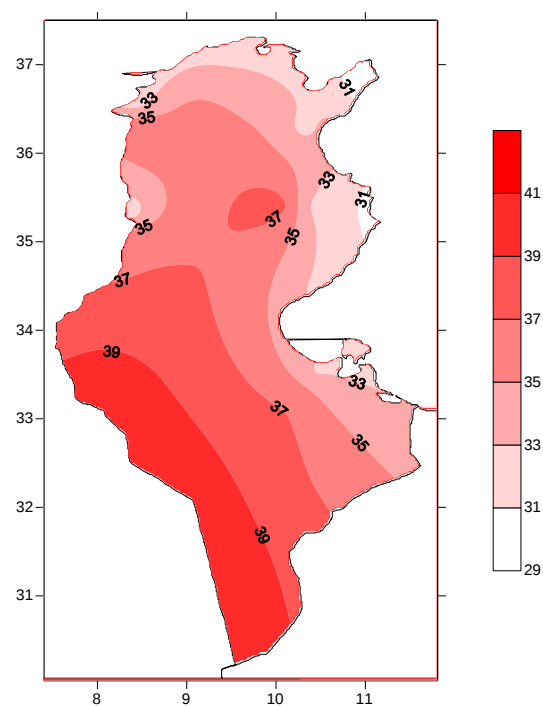
Température maximale moyenne de référence juillet (1981-2010)
