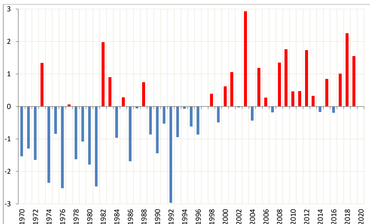
Ecart à la normale 1981-2010 des températures maximales sur les 50 dernières années : Mois de Juillet
