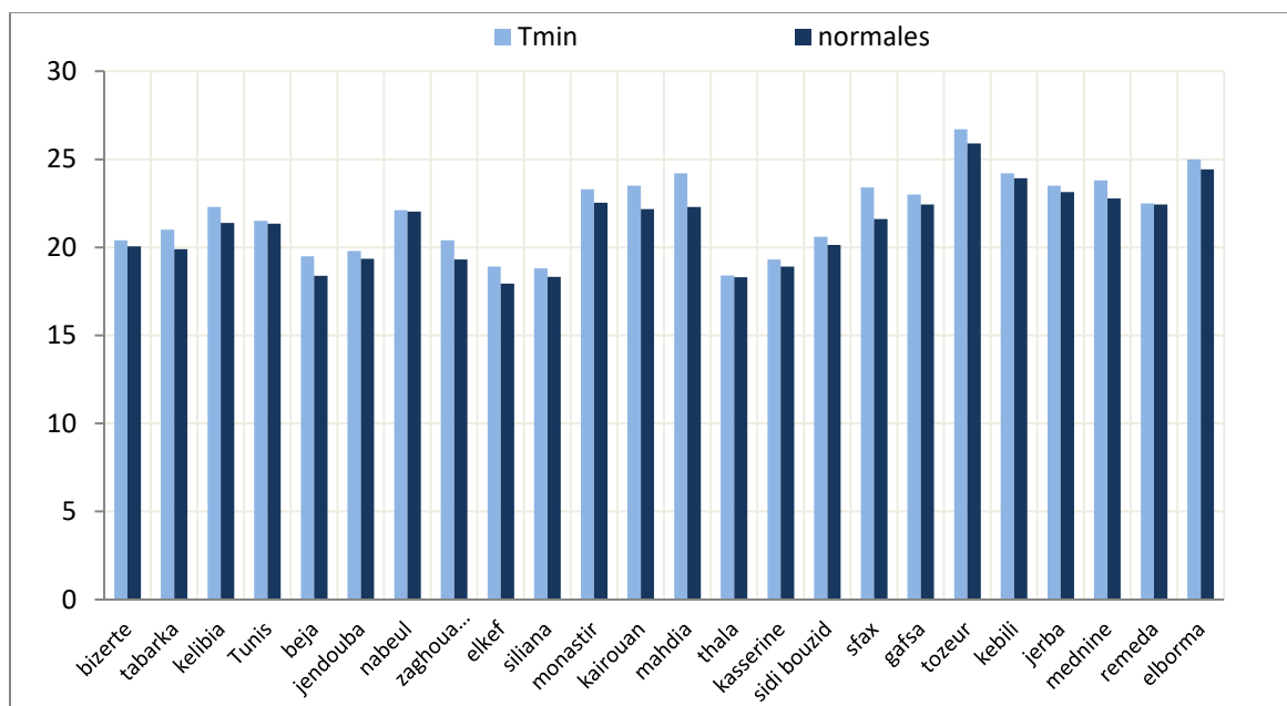
Comparaison des températures minimales aux normales du mois de Juillet
