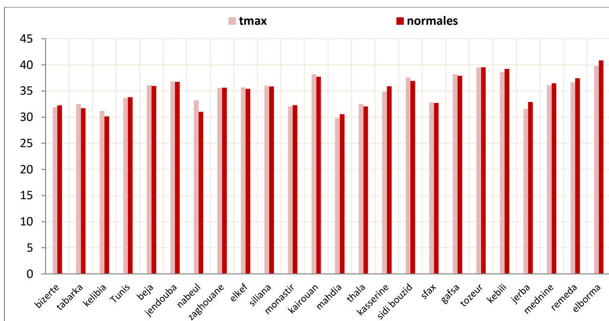
Comparaison des températures maximales aux normales du mois de Juillet
