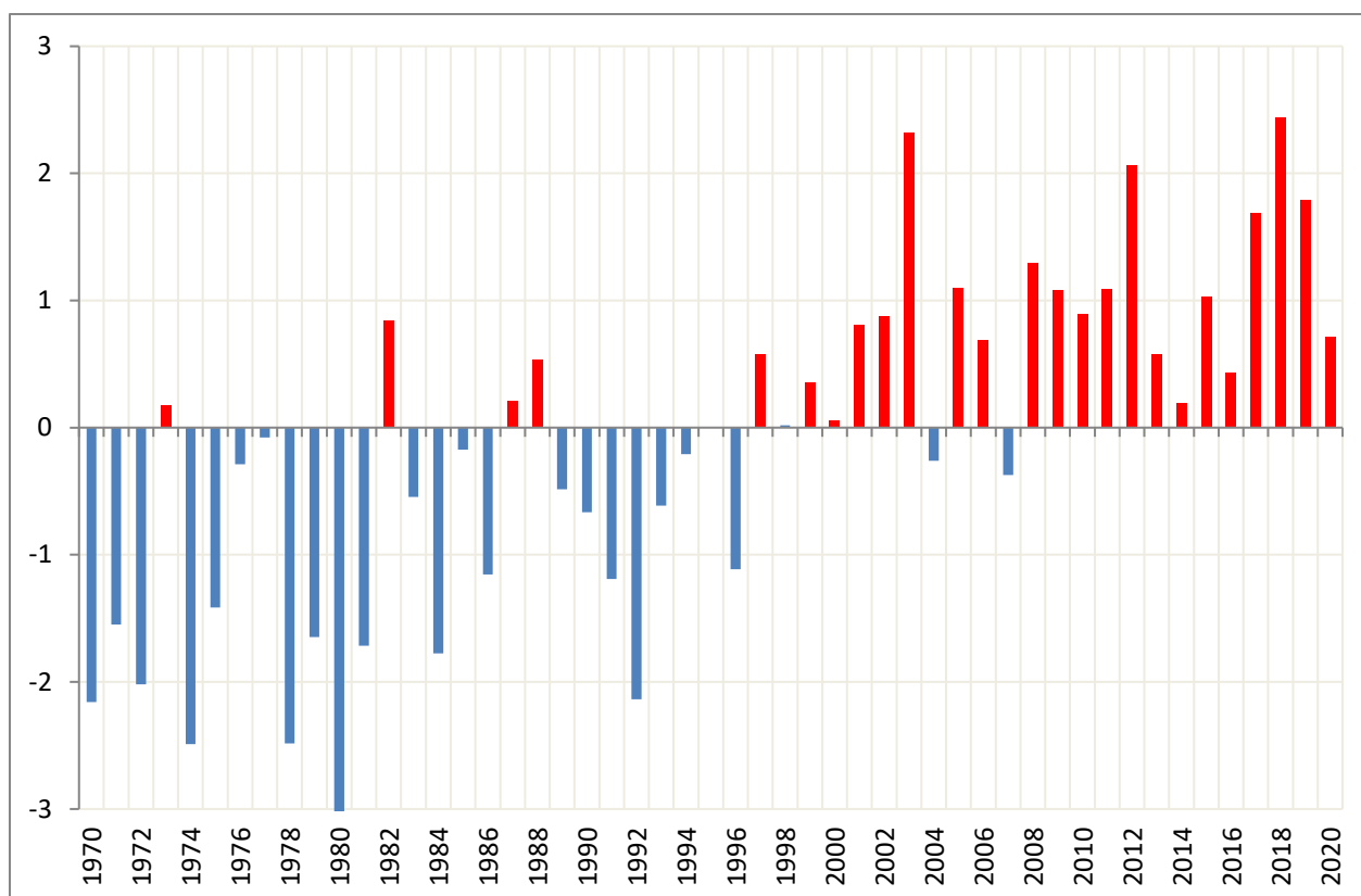
Ecart à la normale 1981-2010 des températures minimales sur les 50 dernières années : Mois de Juillet
