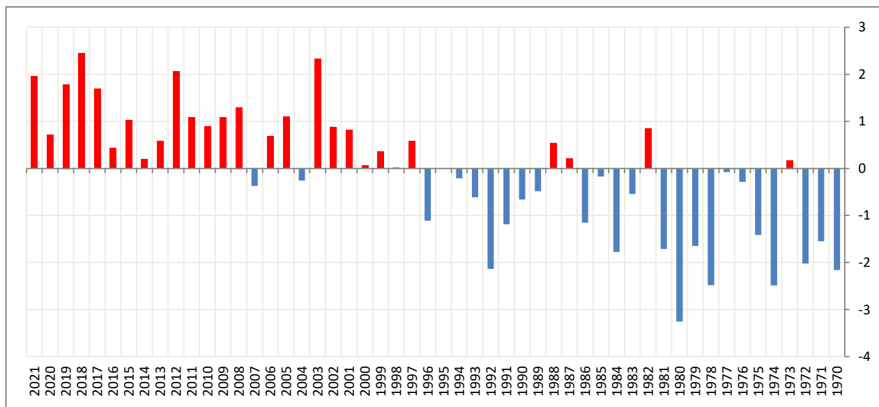
فارق معدّل الحرارة الصغرى خلال شهر جويلية بالنسبة إلى المعدل المرجعي منذ سنة 1970
