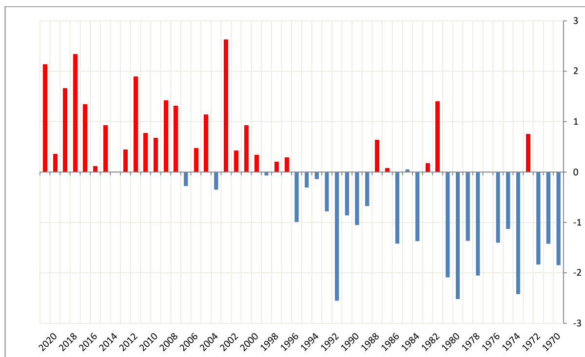
فارق معدل الحرارة المتوسطة لشهر جويلية بالنسبة إلى المعدل الشهري المرجعي منذ سنة 1970
