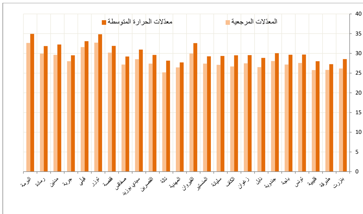
مقارنة معدلات الحرارة المتوسطة لشهر جويلية 2021 بالمعدلات المرجعية (1981-2010)
