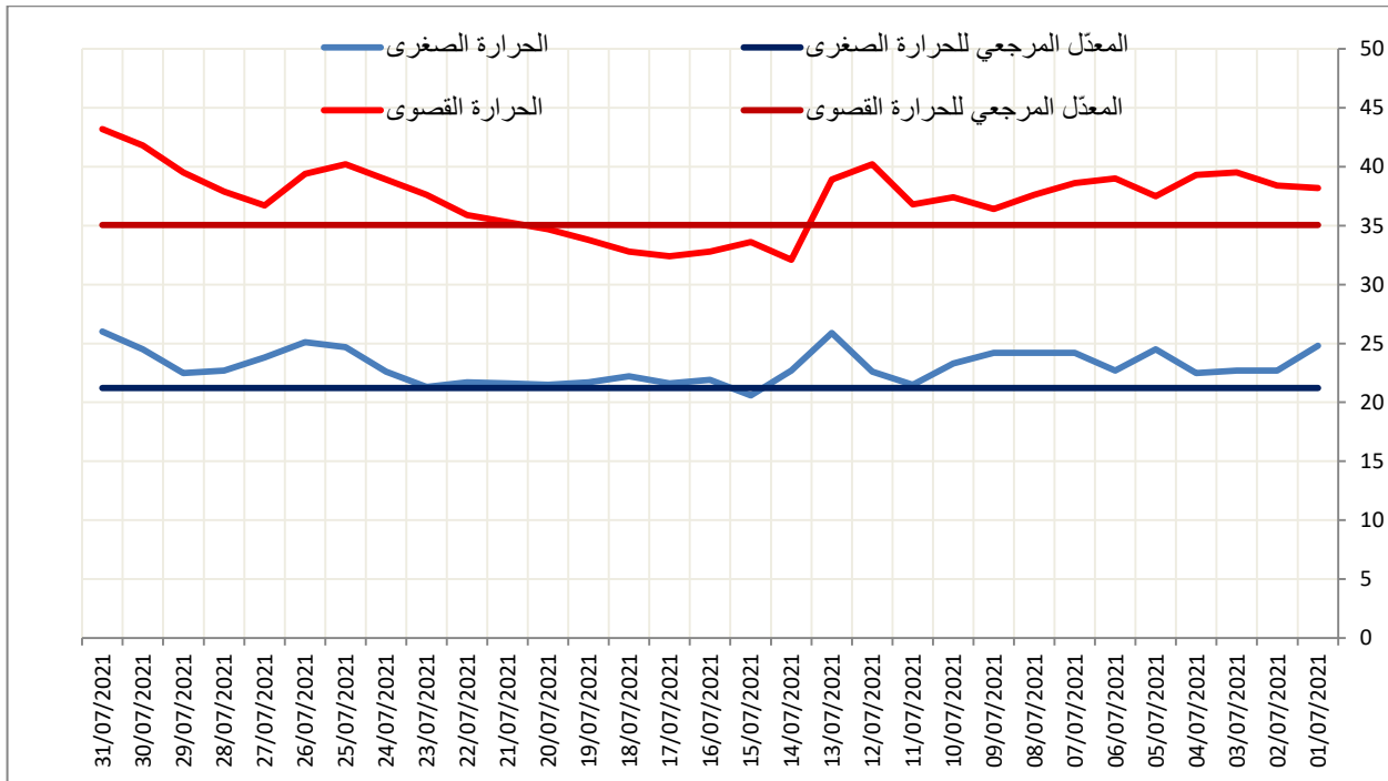
التطور اليومي للحرارة القصوى والصغرى خلال شهر جويلية 2021
