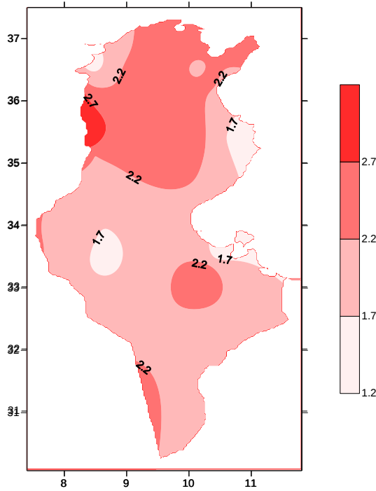
فارق الحرارة المتوسطة بالمعدلات المرجعية
