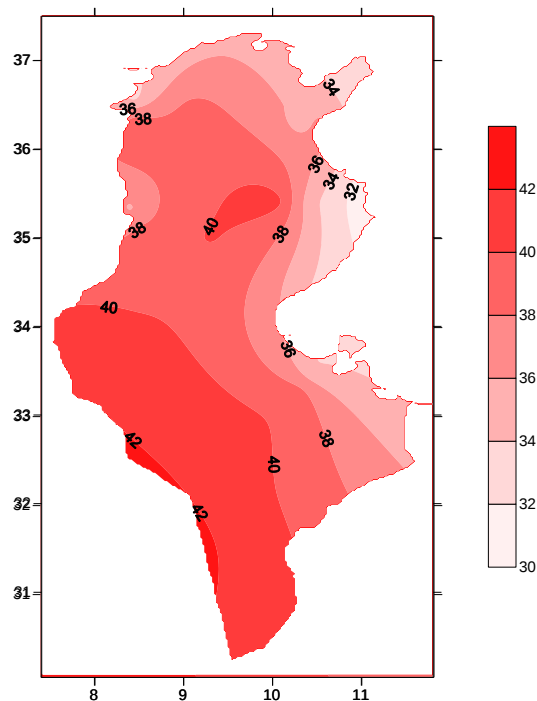
معدل الحرارة القصوى (درجة) لشهر جوان 2021
