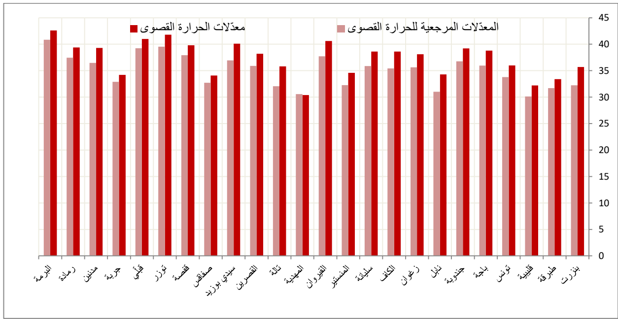
مقارنة معدّلات الحرارة القصوى لشهر جويلية 2021 بالمعدّلات المرجعية (1981-2010)
