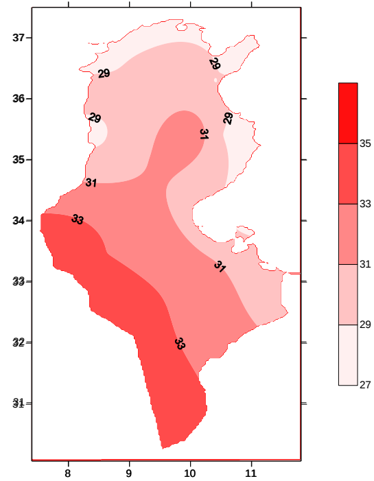
معدل الحرارة المتوسطة (درجة) لشهر جويلية 2021
