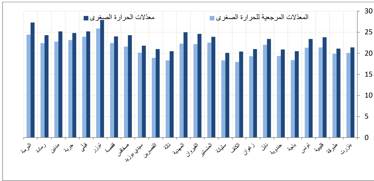
مقارنة معدّلات الحرارة الصغرى لشهر جويلية 2021 بالمعدّلات المرجعية (1981-2010)
