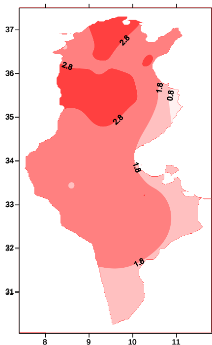
الفارق عن المعدل المرجعي
