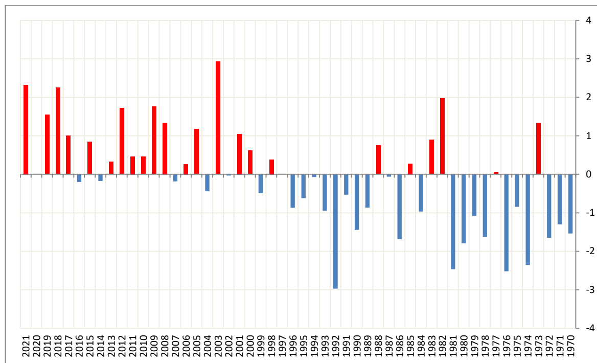
فارق معذل الحرارة القصوى لشهر جويلية بالنسبة إلى المعدل المرجعي (1981 - 2010) منذ سنة 1970
