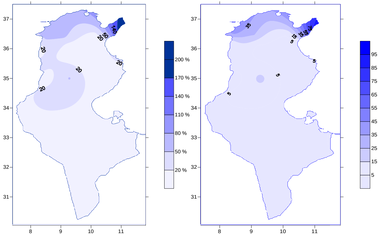
نسبة مجموع أمطار شهر سبتمبر 2021 إلى المجموع الشهري المرجعي
