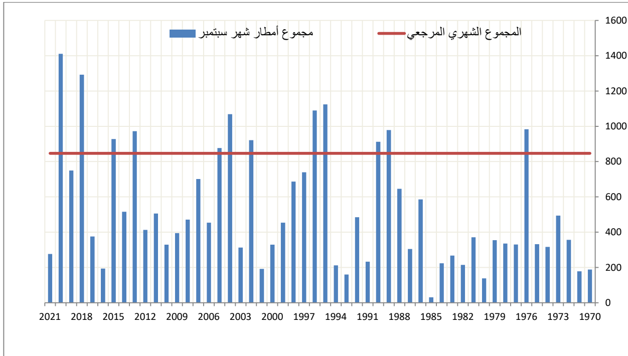
مجموع الأمطار (بحساب المليمتر) بكافة المحطات الرئيسة لشهر سبتمبر منذ سنة 1970
