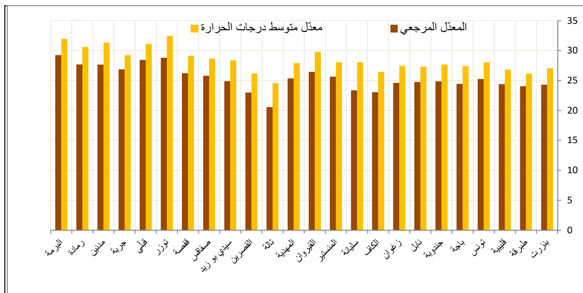
مقارنة معدّلات متوسط درجات الحرارة لشهر سبتمبر 2021 بالمعدّلات المرجعية ( 1981 - 2010 )
