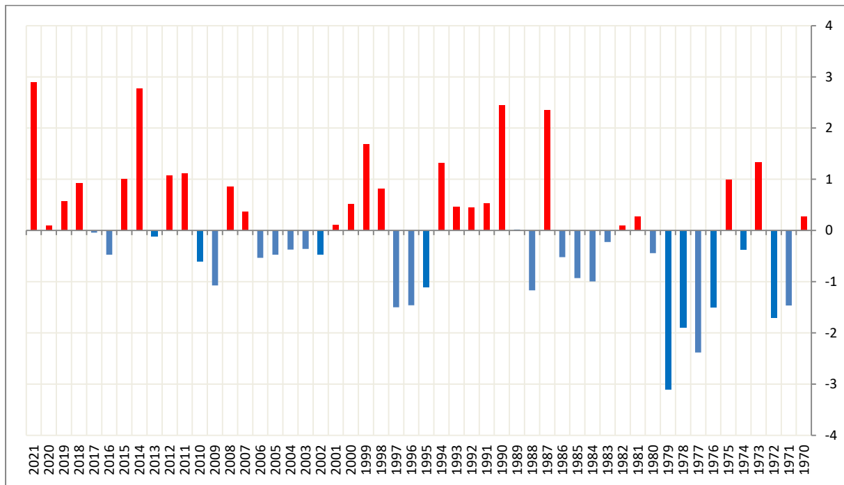
فارق معدّل الحرارة القصوى لشهر سبتمبر بالنسبة إلى المعدل المرجعي منذ سنة 1970
