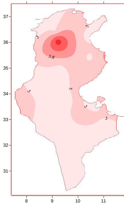
فارق معدل الحرارة القصوى بالمعدلات المرجعية
