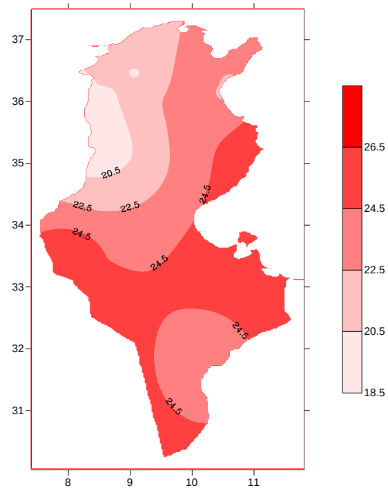
معدل الحرارة الصغرى ( درجة) لشهر سبتمبر 2021
