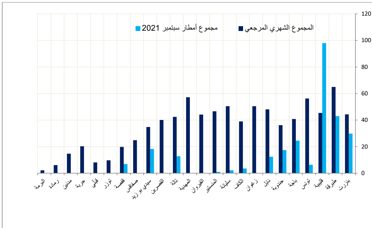
مقارنة مجموع كميات الأمطار ( بحساب المليمترا ) لشهر سبتمبر 2021 بالمجموع المرجعي
