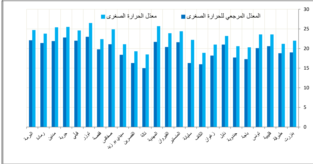
مقارنة معدّلات الحرارة الصغرى لصيف 2021 بالمعدّلات المرجعية (1981-2010)
