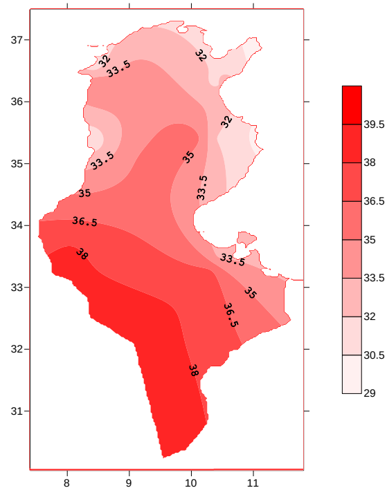
معدّل الحرارة القصوى (درجة) لشهر سبتمبر 2021
