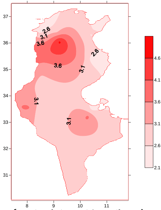
فارق معدّل متوسط الحرارة بالمعدّلات المرجعية
