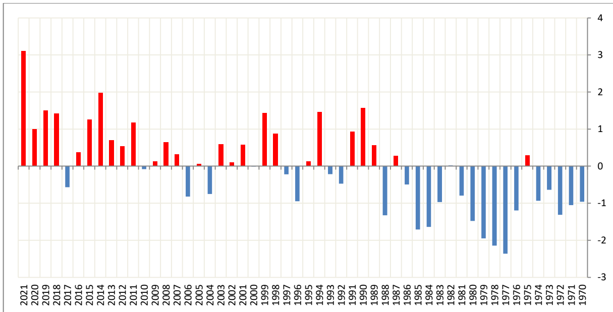
فارق معدّل الحرارة الصغرى لشهر سبتمبر بالنسبة إلى المعدّل المرجعي منذ سنة 1970
