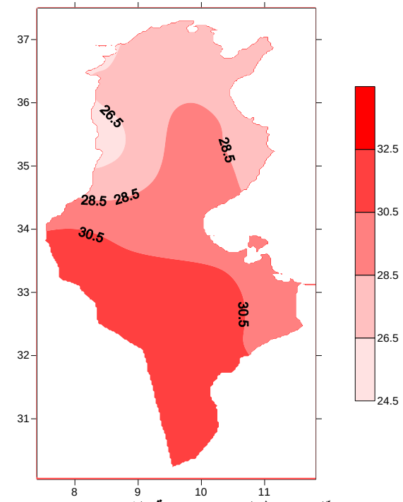
معدّل متوسط الحرارة ( درجة ) لشهر سبتمبر 2021
