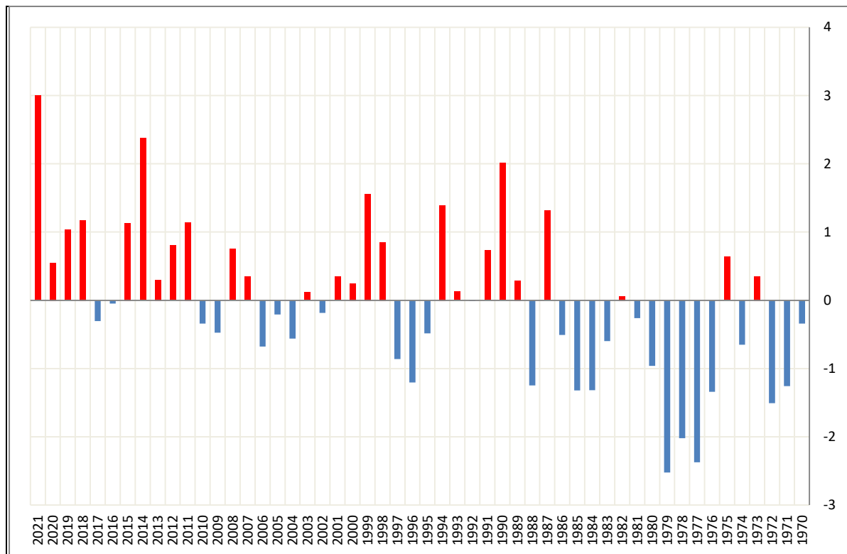
فارق معدّل متوسط درجات الحرارة خلال شهر سبتمبر بالنسبة إلى المعدل المرجعي منذ سنة 1970
