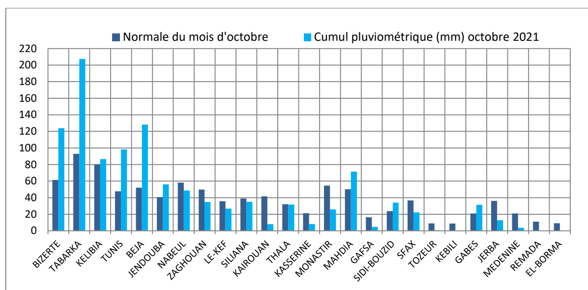
Comparaison des cumuls mensuels des précipitations d'octobre 2021 par rapport aux normales de référence
