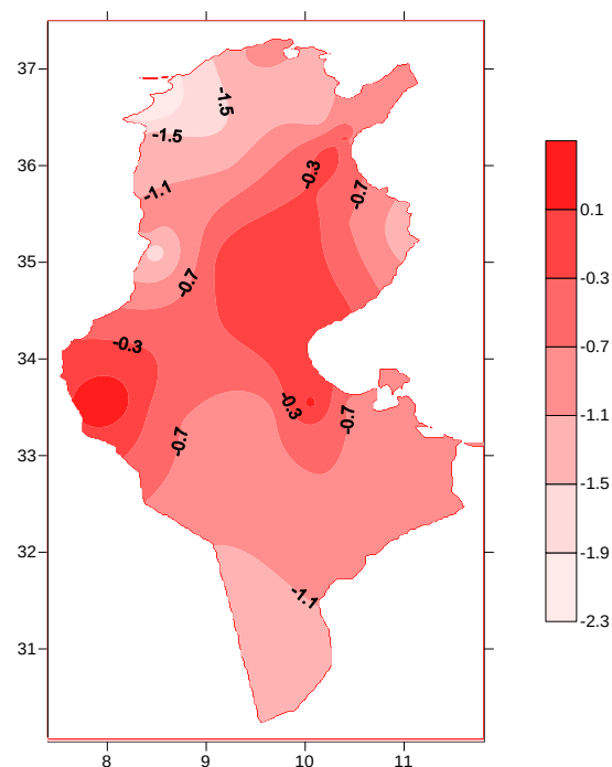
Ecart à la normale de Tmax en (°C)
