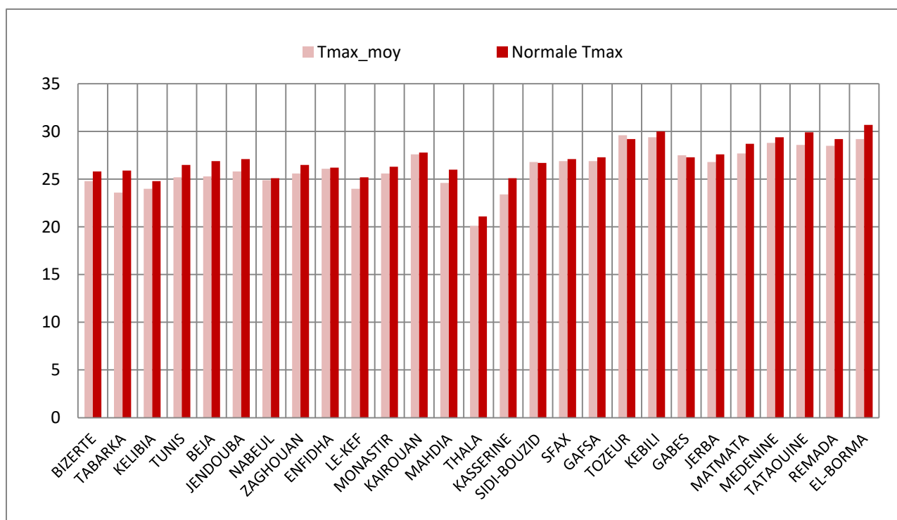
Comparaison des températures maximales ( Octobre 2021) aux normales du mois
