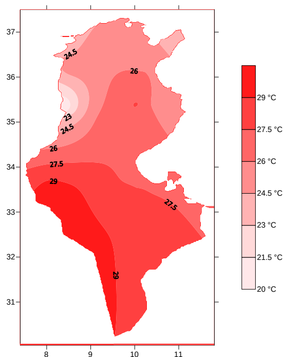
Température maximale (°C) Octobre 2021
