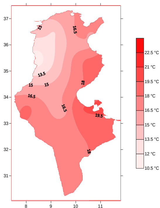
Température minimale (°C) Octobre 2021
