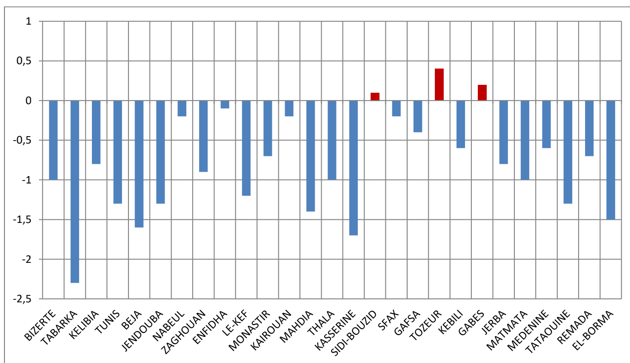
Ecart à la normale (1981-2010) des températures maximales depuis 1970 : Mois d'Octobre
