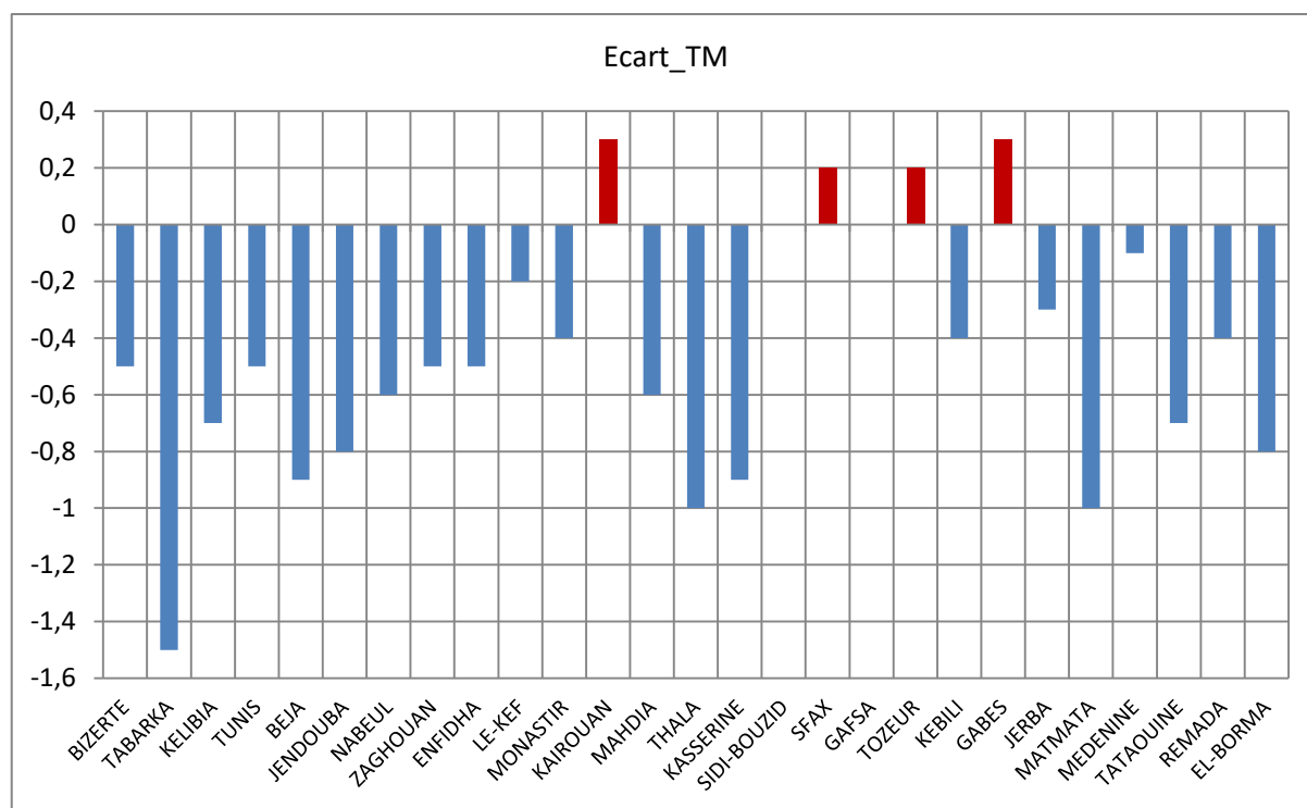
Ecart à la normale (1981-2010) des températures moyennes depuis 1970 : Mois d'octobre
