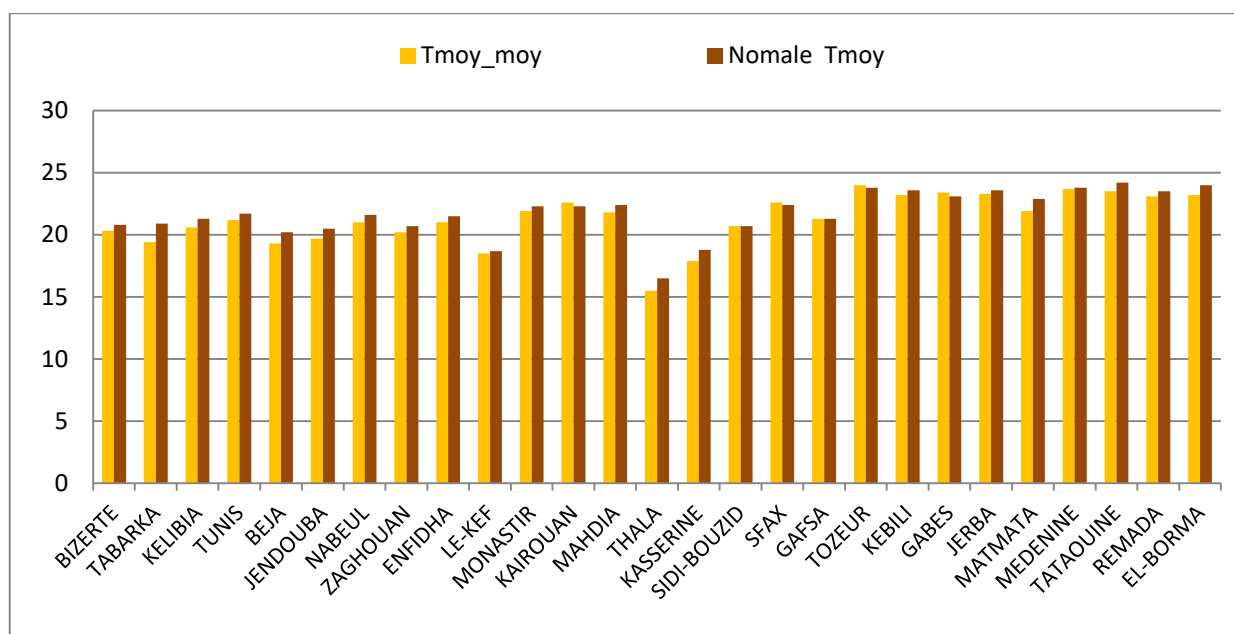
Comparaison des températures moyennes (octobre 2021) aux normales du mois
