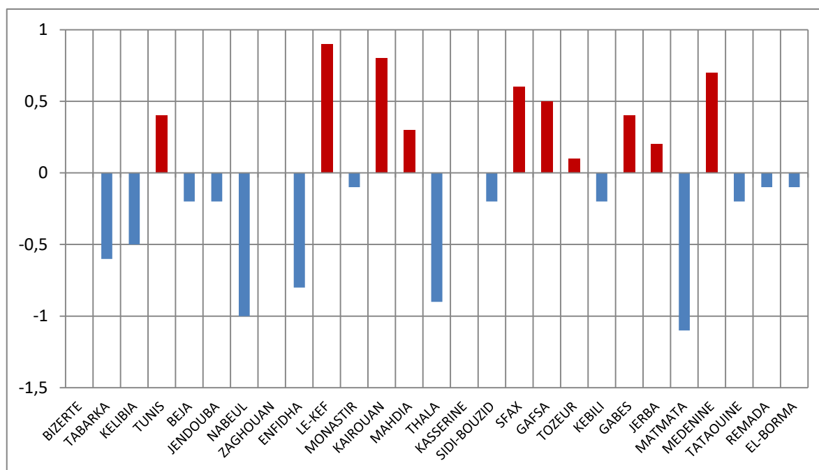
Ecart à la normale des températures minimales sur la période (1970-2021) : Mois d'octobre
