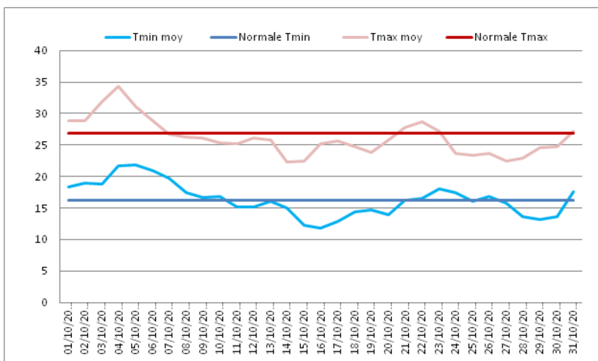
Evolutions des températures quotidiennes en Tunisie par rapport à la normale du mois d'octobre
