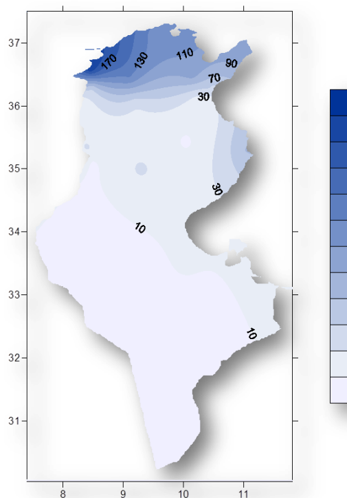
Cumul mensuel (mm) Octobre 2021
