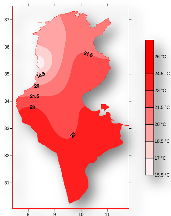
Température moyennne (°C) Octobre 2021
