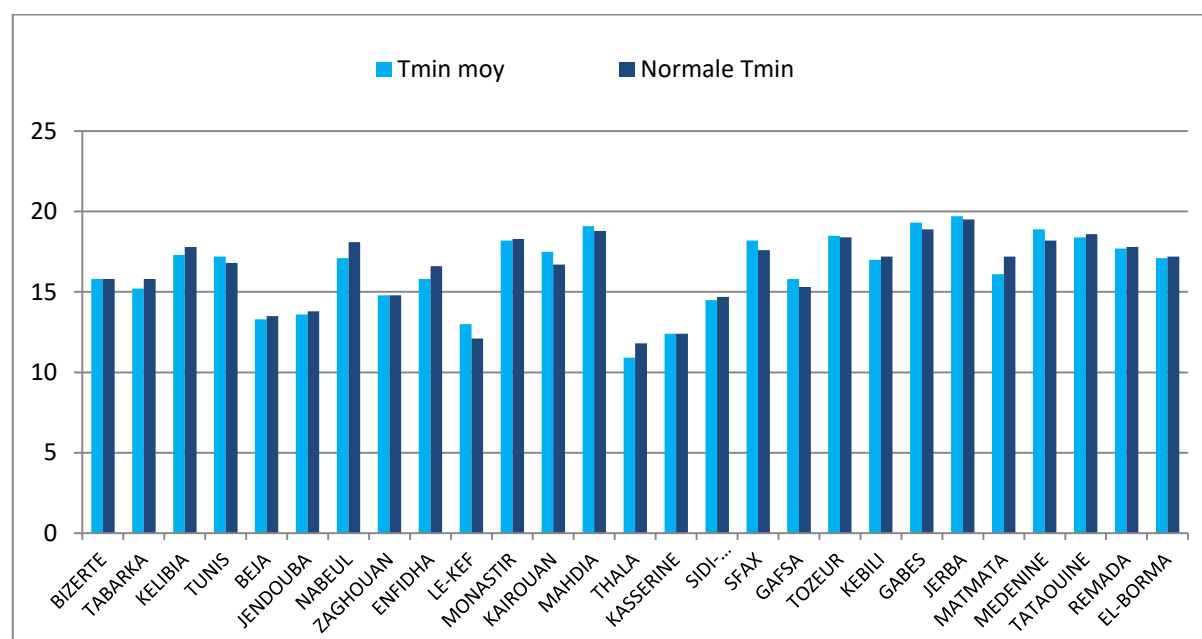
Comparaison des températures minimales (octobre 2021) aux normales du mois
