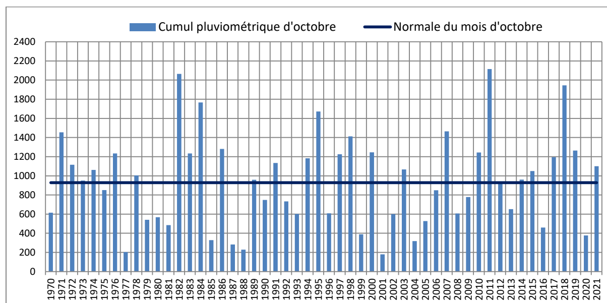
Cumul mensuel des précipitations sur la période (1970-2021) en Tunisie: Mois d'octobre
