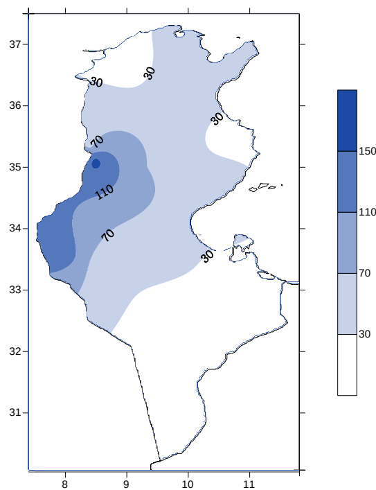
Rapport à la normale (%)
