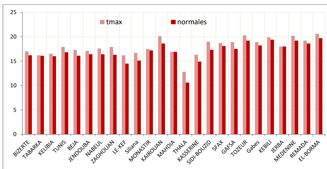
Comparaison des températures maximales aux normales du mois de Février
