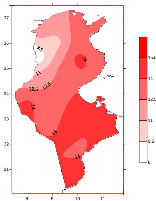
Température moyenne (°C)
