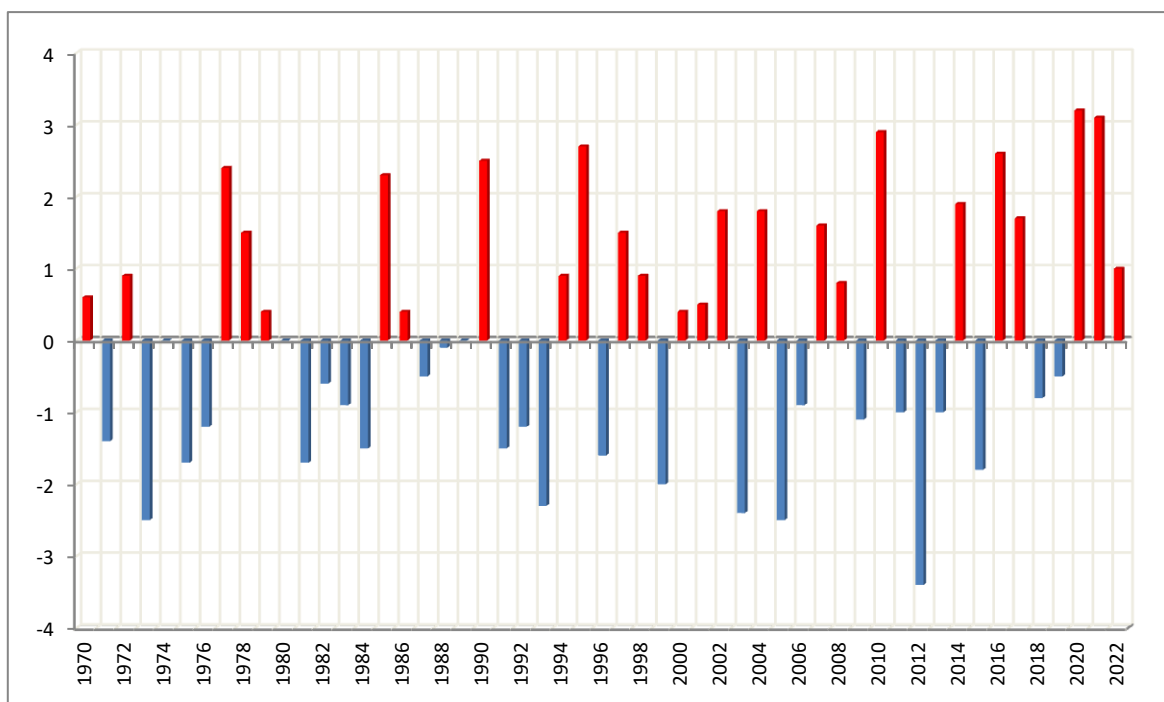
Ecart à la normale 1981-2010 des températures maximales depuis 1970 : Mois de Février
