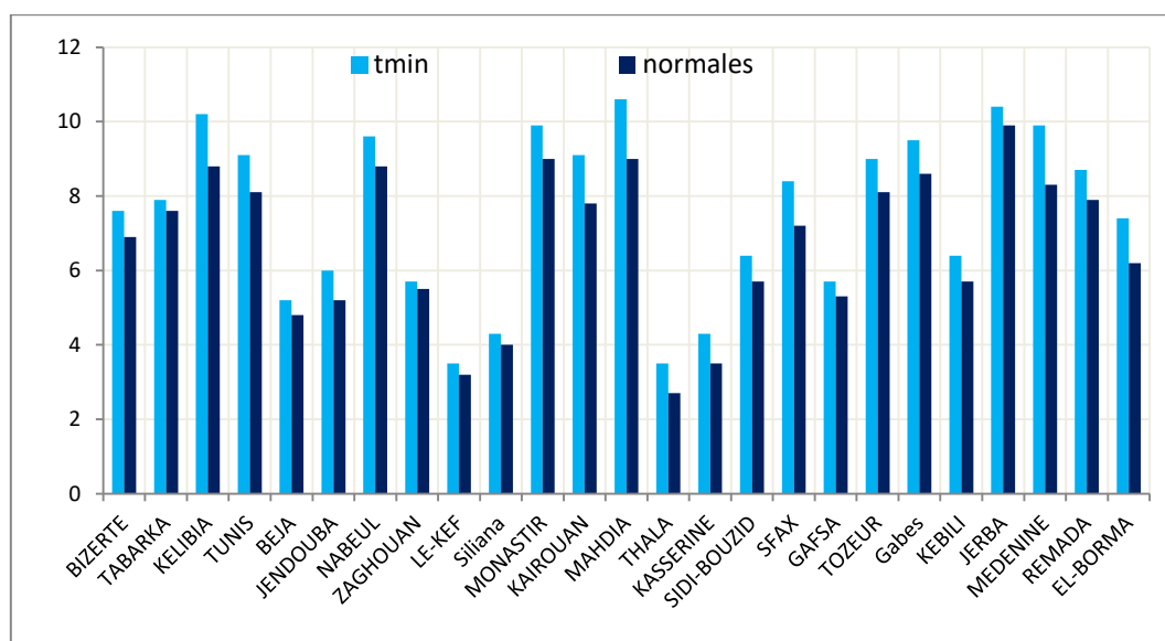
Comparaison des températures minimales aux normales du Mois de Février
