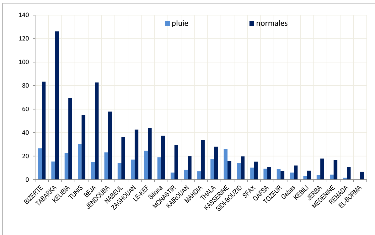
Comparaison des cumuls mensuels des précipitations par rapport aux normales de référence des cumuls
