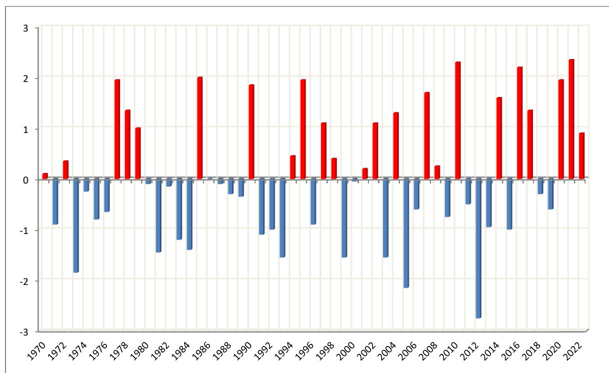
Ecart à la normale 1981-2010 des températures moyennes depuis 1970 : Mois de Février
