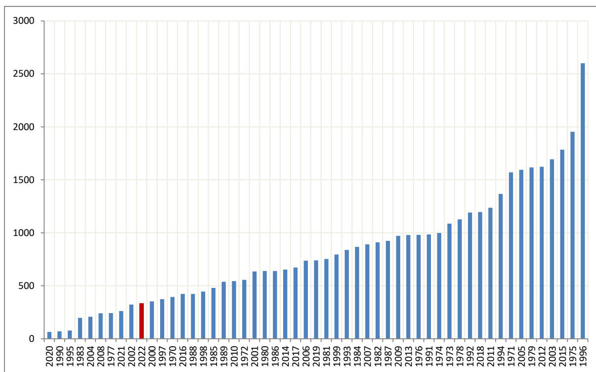
Classement des cumuls mensuels des précipitations (mois de Février)
