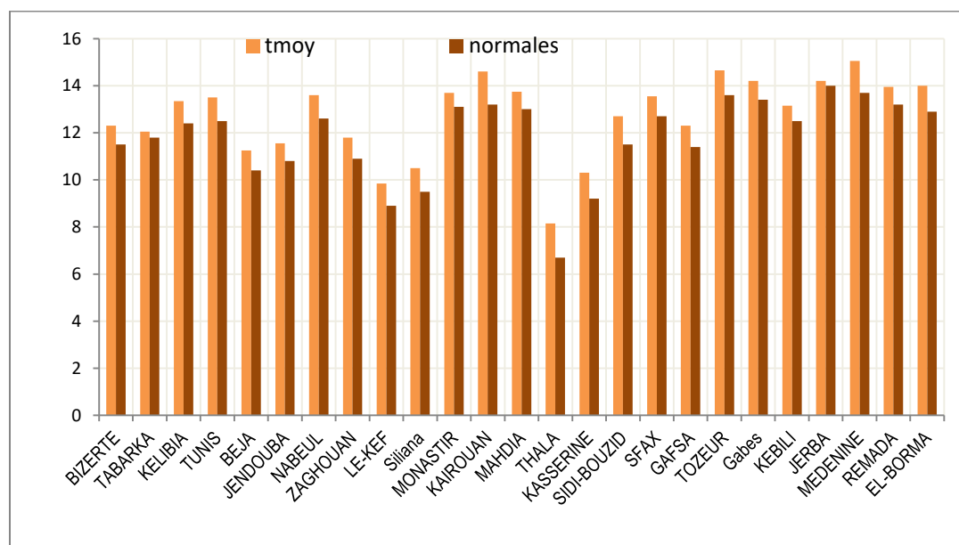
Comparaison des températures moyennes aux normales du mois de Février
