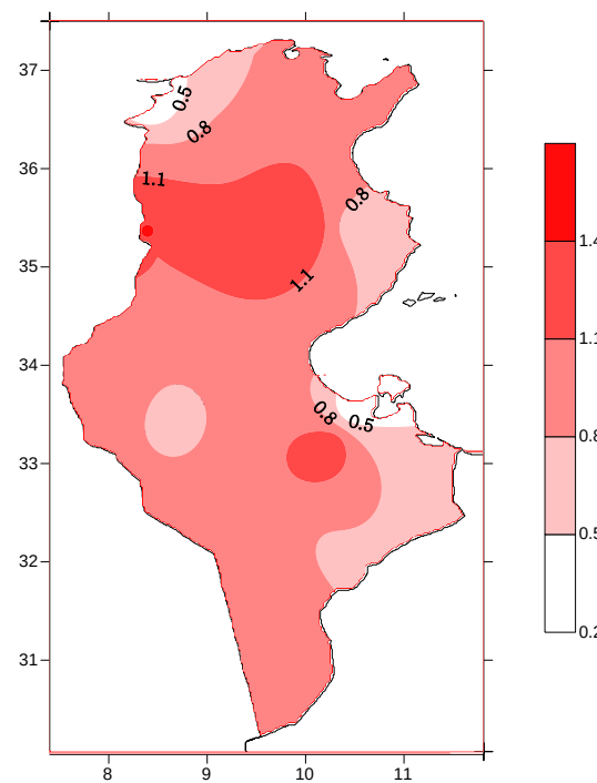
Ecart de Tmoy à la normale (°C)
