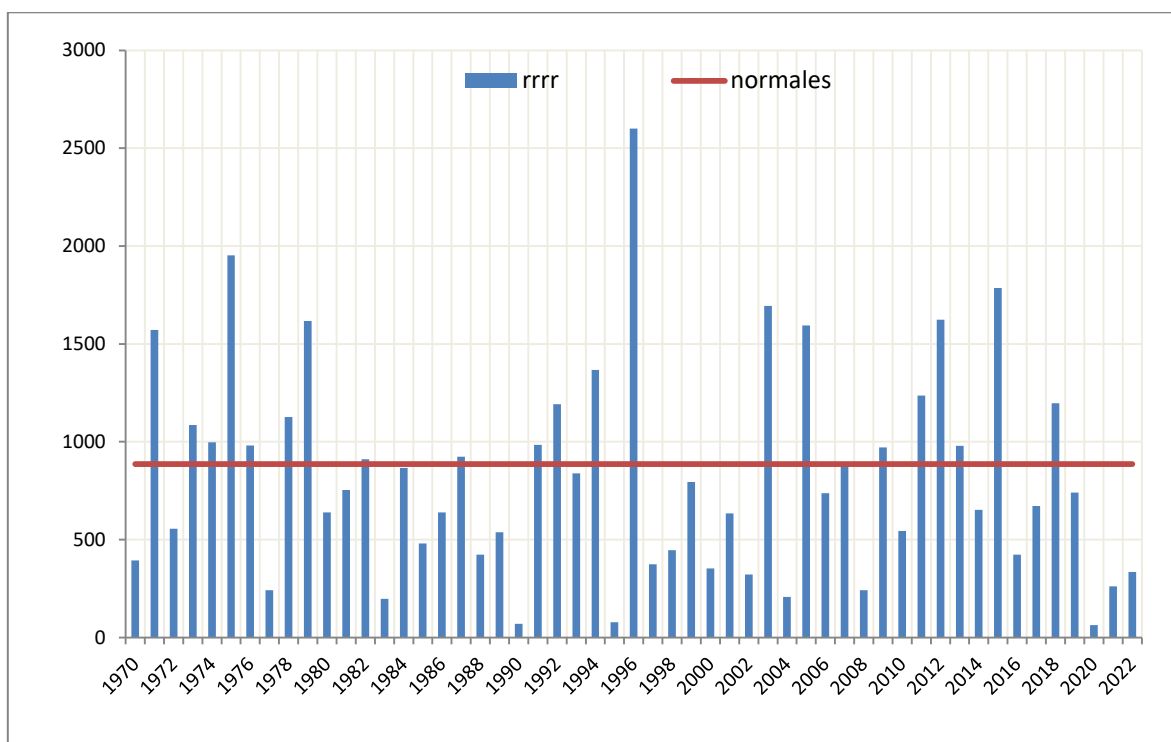
Cumul mensuel des précipitations depuis 1970 sur la Tunisie: Mois de Février
