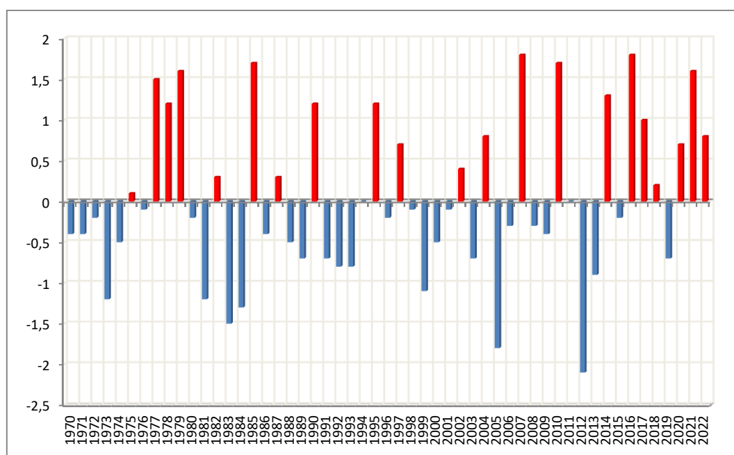
Ecart à la normale 1981-2010 des températures minimales depuis 1970 : Mois de Février
