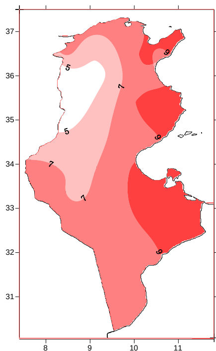
Température minimale en (°C)
