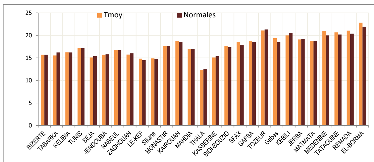
Comparaison des températures moyennes aux normales du Mois d'Avril
