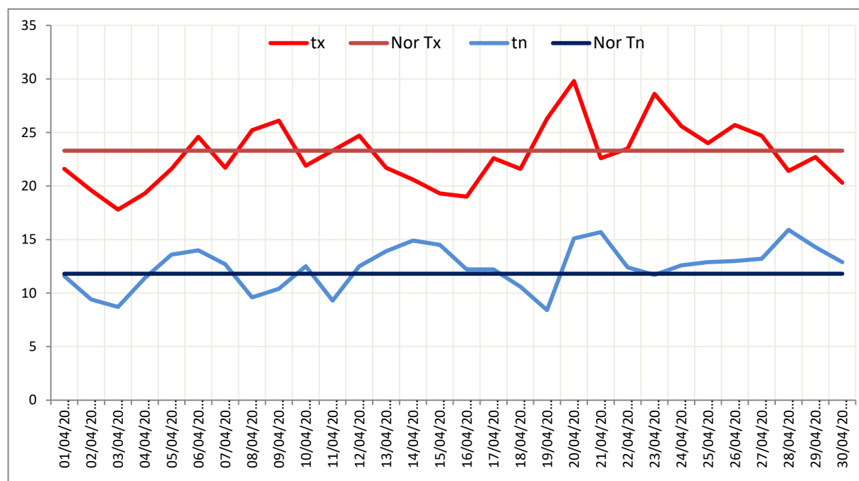
Evolution quotidienne des températures au cours du mois d'avril 2022 par rapport aux moyennes de référence
