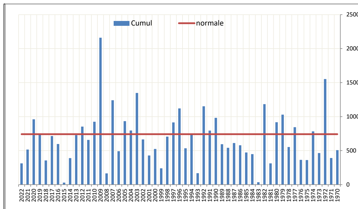
Pluie (mm) des stations principales pour le mois d'Avril depuis 1970
