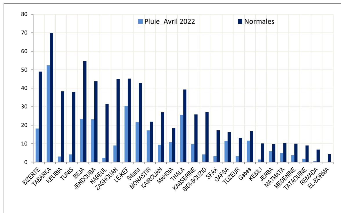
Comparaison des quantités de pluie (mm) du mois d'avril 2022 avec la normale (1991-2020)
