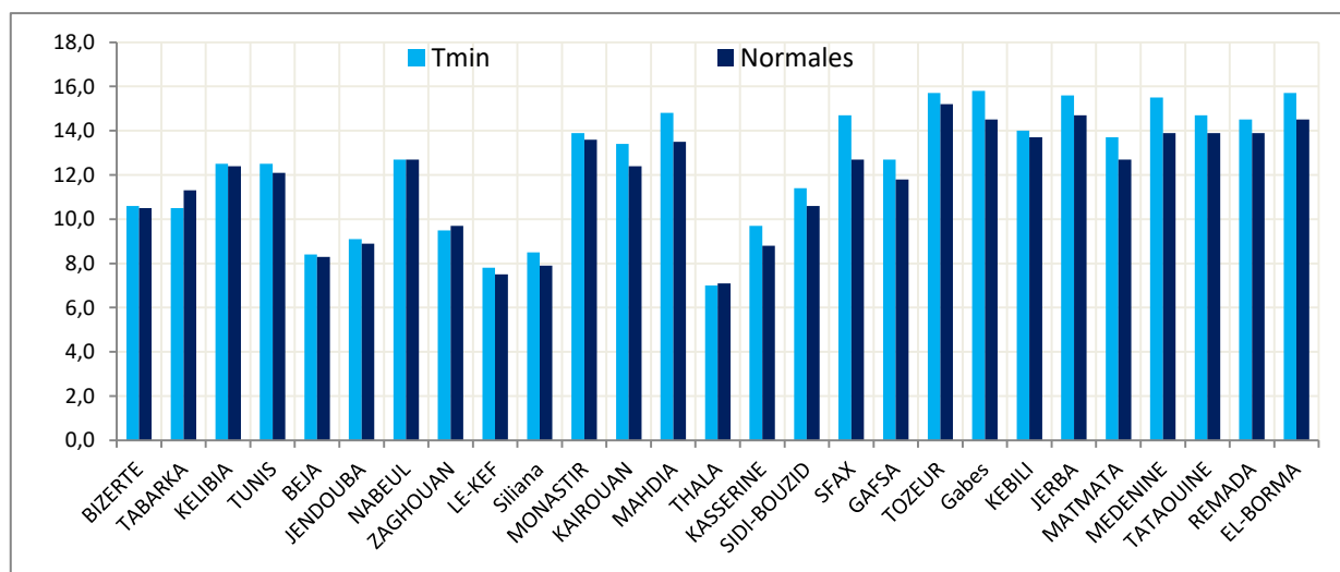
Comparaison des températures minimales aux normales du Mois d'Avril
