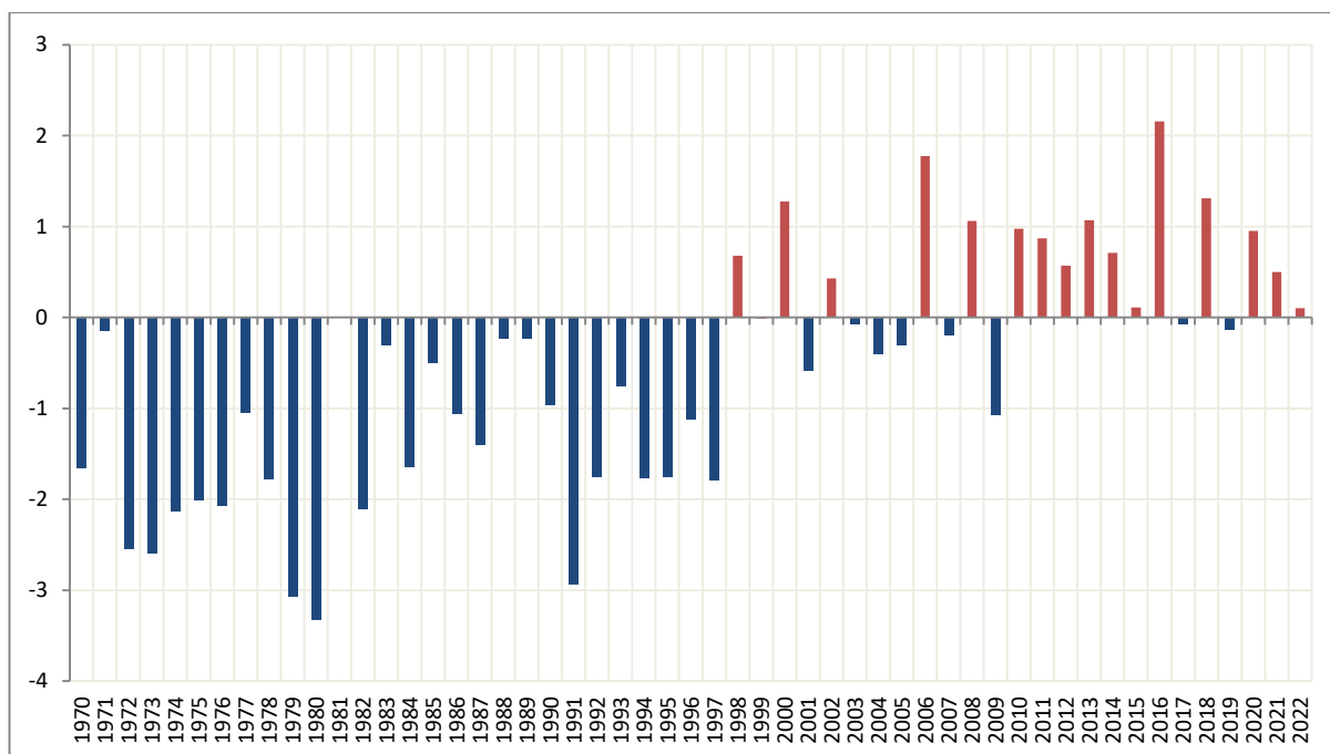
Écart à la normale 1991-2020 des températures moyennes depuis 1970 : Mois d'Avril
