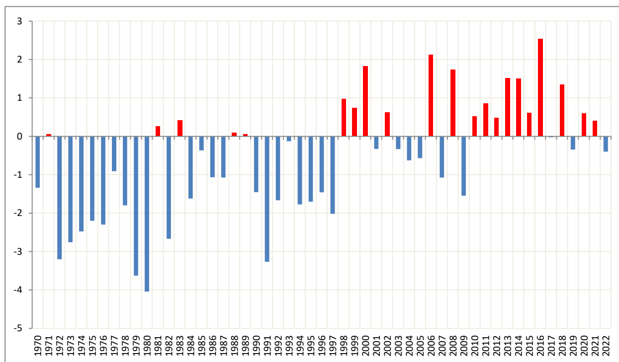
Ecart à la normale 1991-2020 des températures maximales depuis 1970 : Mois d'Avril
