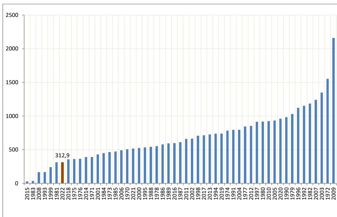
Classement des cumuls de pluie du mois d'avril sur la période (1970-2022)
