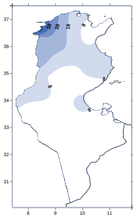
Cumul de pluie aux stations principales
