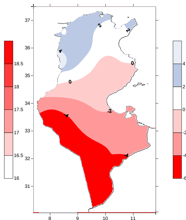
Écart à la normale de Tmoy
