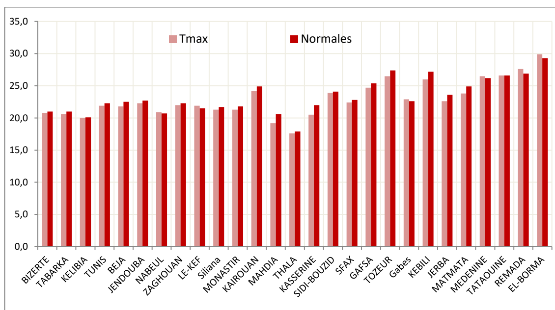
Comparaison des températures maximales aux normales du Mois d'Avril
