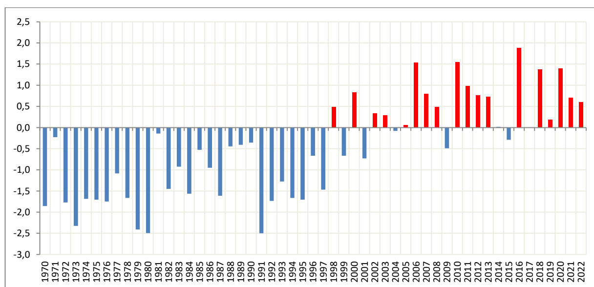
Écart à la normale (1991-2020) des températures minimales depuis 1970 : Mois d'Avril
