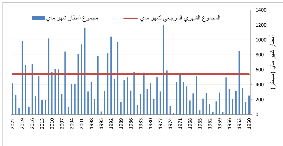
مجموع الأمطار (بحساب المليمتر) بكافة المحطات الرئيسية لشهر ماي منذ سنة 1950
