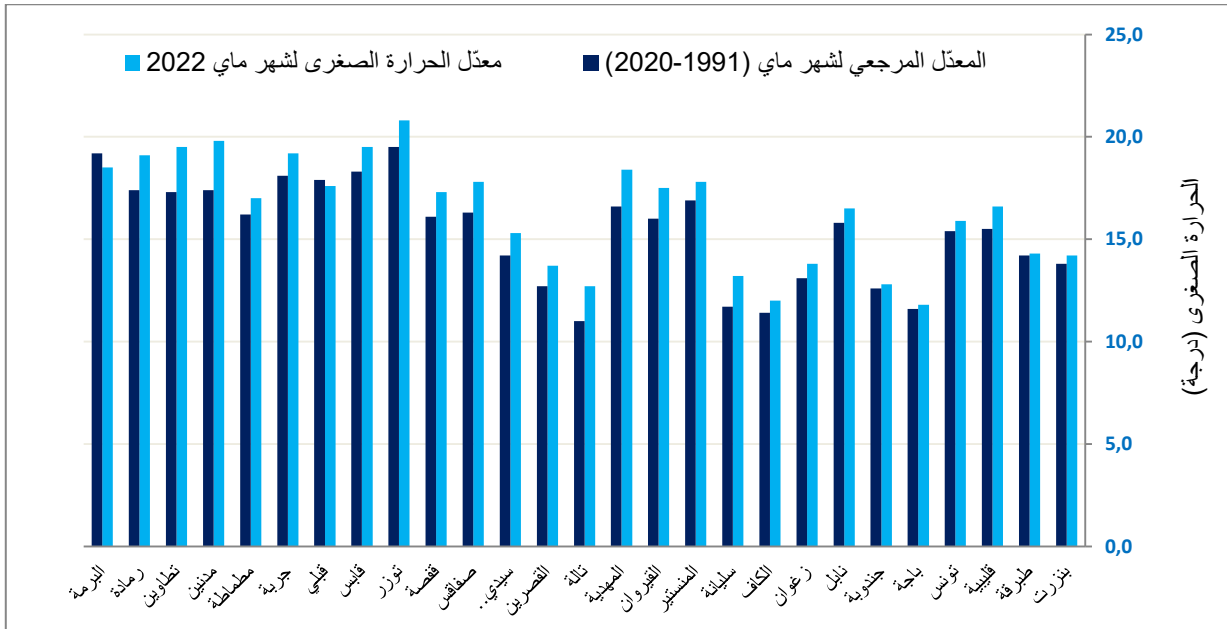
مقارنة معدّل الحرارة الصغرى لشهر ماي 2022 بالمعدّلات المرجعية (1991 - 2020)
