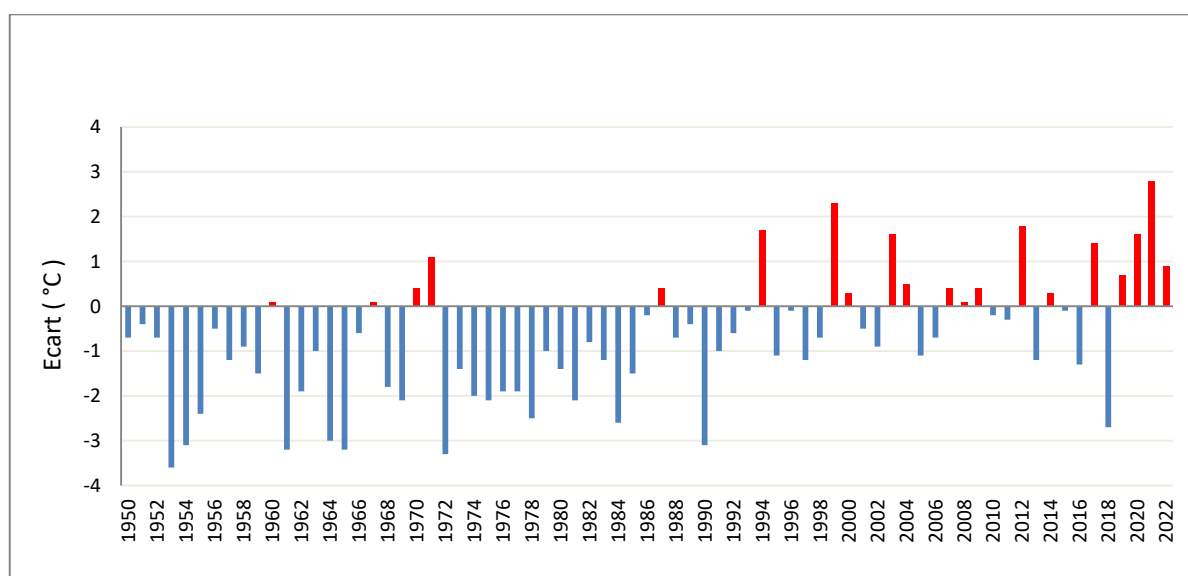
Ecart à la normale 1991-2020 des températures maximales depuis 1950 : Mois d'Aout
