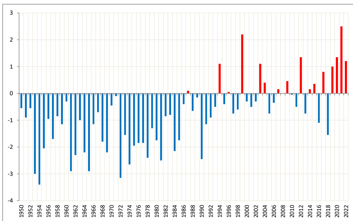
Ecart à la normale 1991-2020 des températures moyennes depuis 1950 : Mois d'Aout
