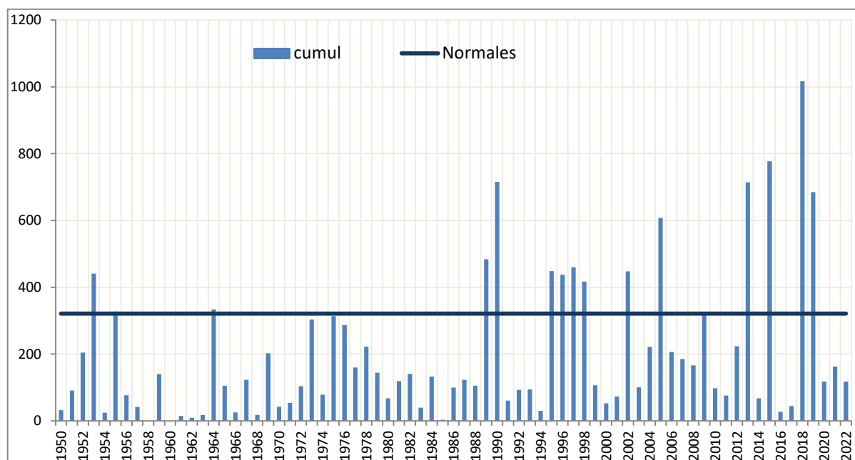
Cumul mensuel des précipitations depuis 1950 sur la Tunisie: Mois d'Aout
