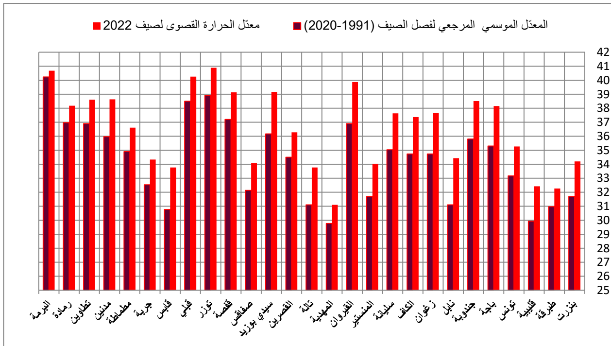
مقارنة المعدلات الموسمية للحرارة القصوى لفصل الصيف بالمعدلات المرجعية (2020-1991)
