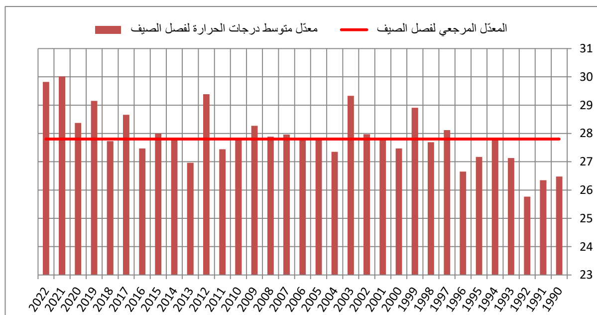
معدّل متوسط درجات الحرارة لفصل الصيف منذ سنة 1990 إلى سنة 2022
