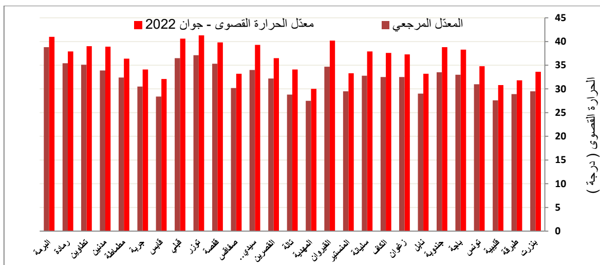
مقارنة بين معدلات الحرارة القصوى لشهر جوان 2022 بالمعدلات المرجعية (1991-2020)
