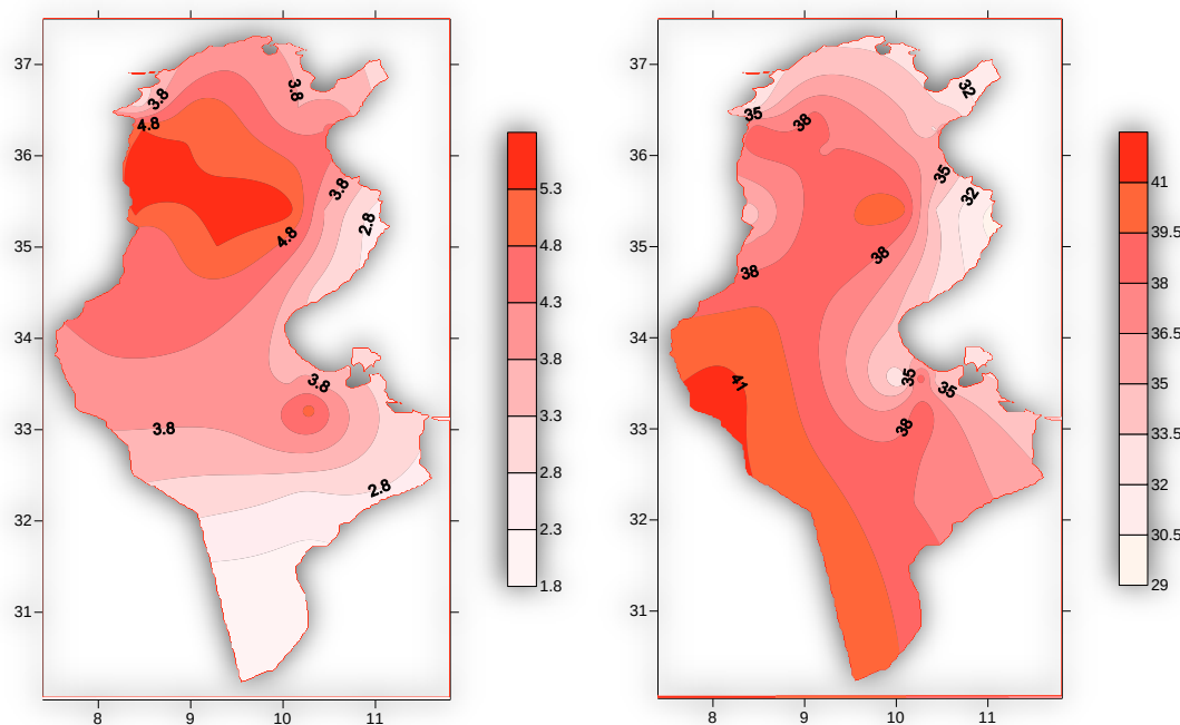
الفارق بين الحرارة القصوى و المعدل المرجعي (درجة)
