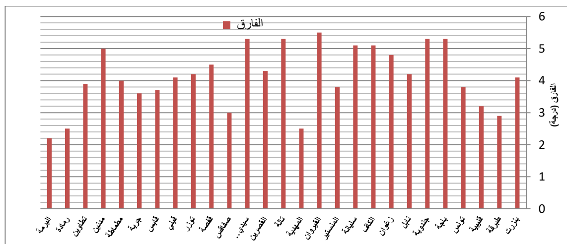
فارق معدلات الحرارة القصوى لشهر جوان 2022 عن المعدلات المرجعية (1991 - 2020)
