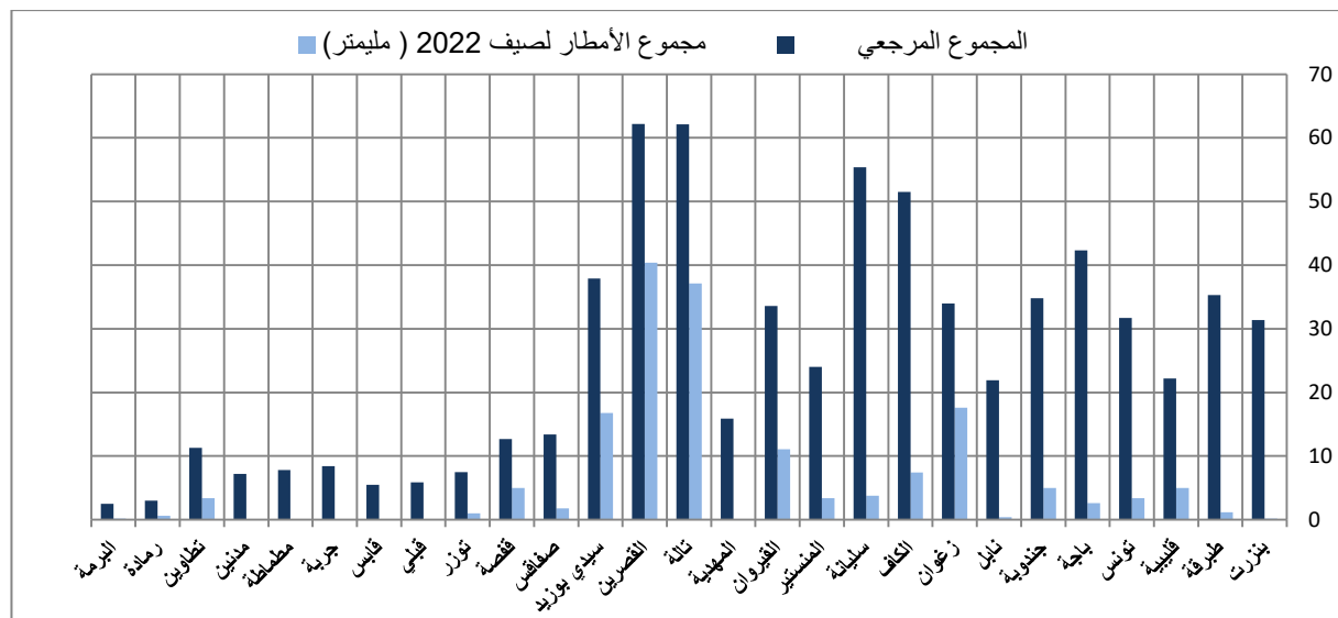
مقارنة مجموع الأمطار لصيف 2022 بالمجموع الموسمي المرجعي (1991-2020) حسب المحطات
