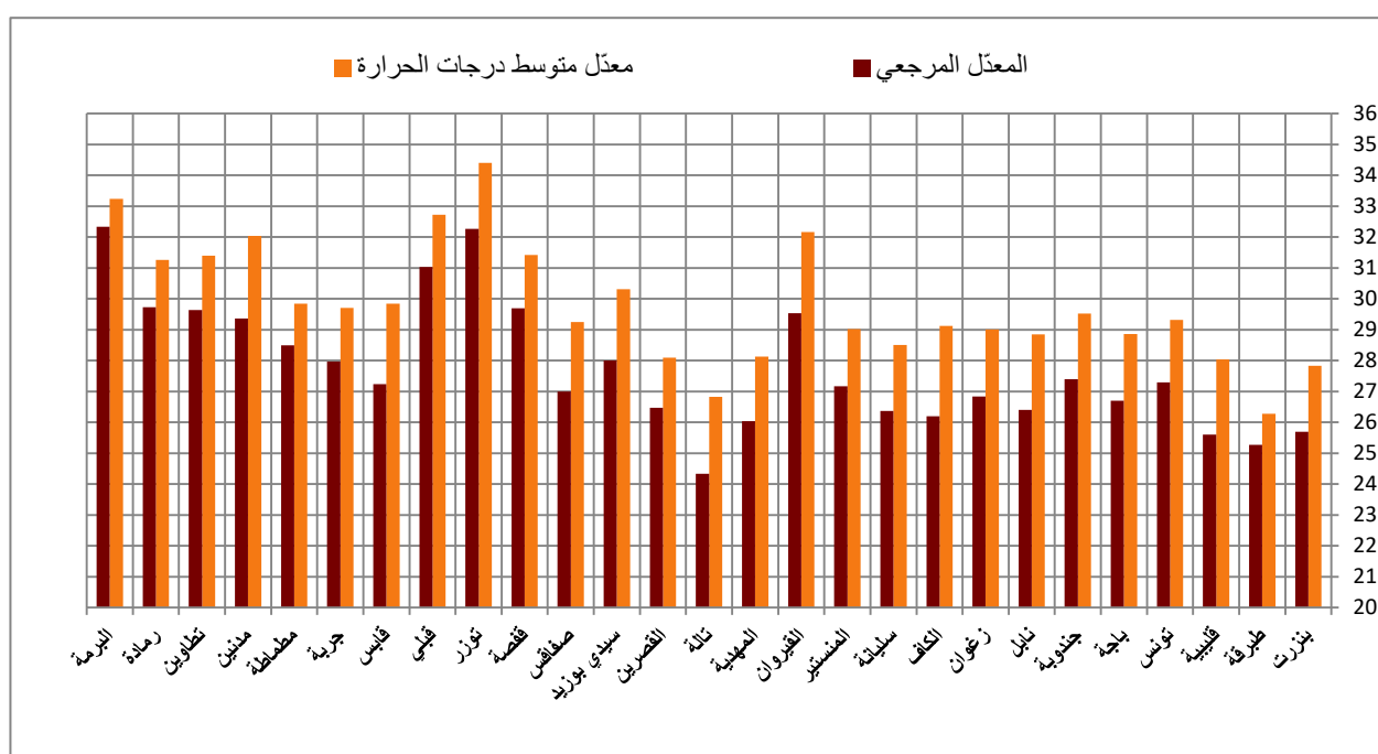
مقارنة معدّلات متوسط درجات الحرارة لصيف 2022 بالمعدّلات المرجعية (1991-2020)
