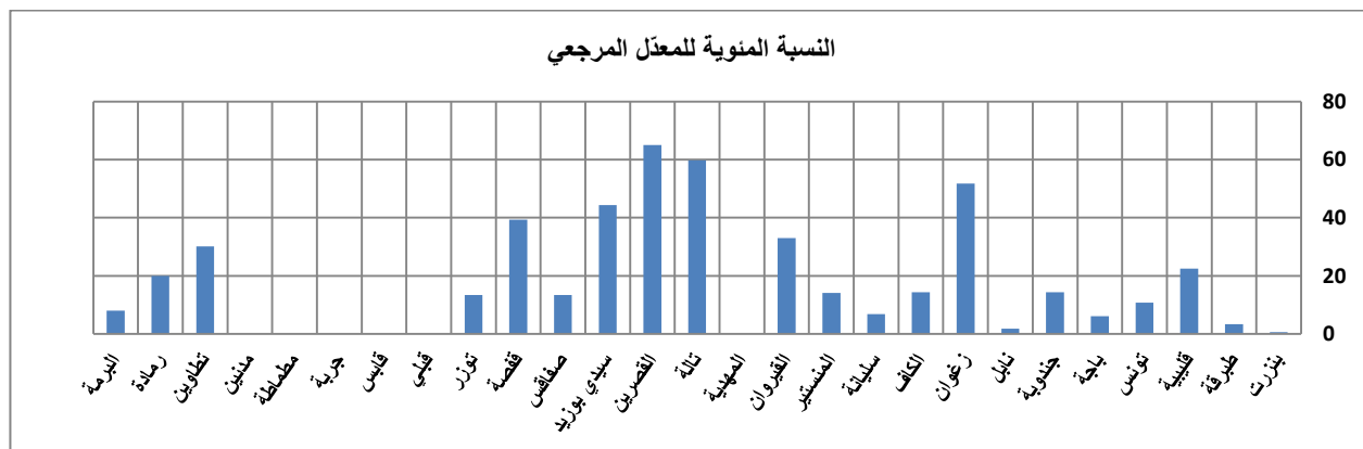
النسبة المئوية لمجموع الأمطار لفصل الصيف بالمجموع الموسمي المرجعي (1991-2020) حسب المحطات
