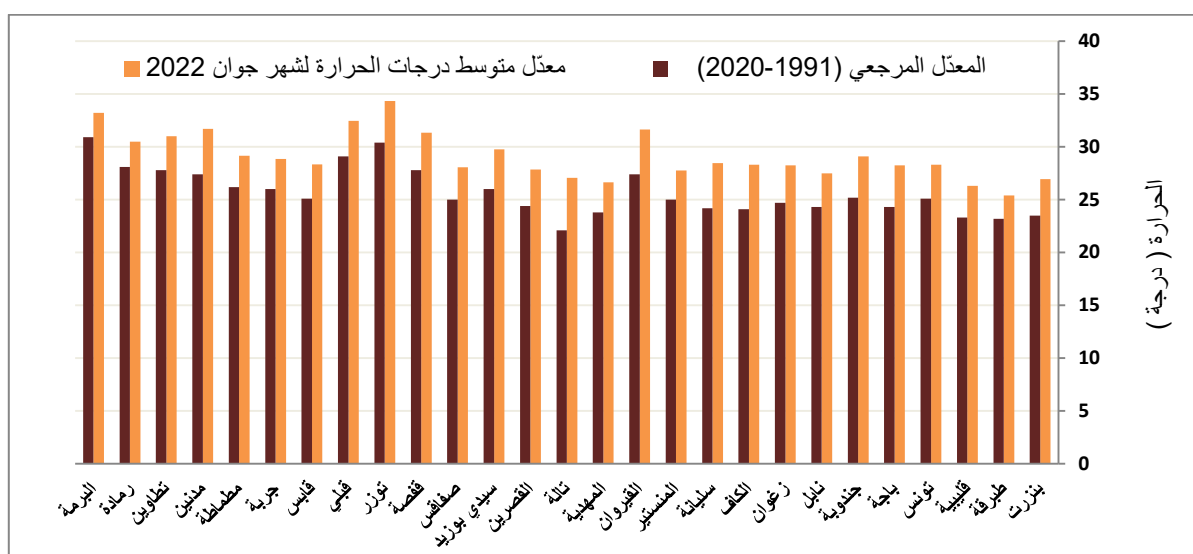
مقارنة معدّلات متوسط درجات الحرارة لشهر جوان بالمعدّلات المرجعية (1991-2020)
