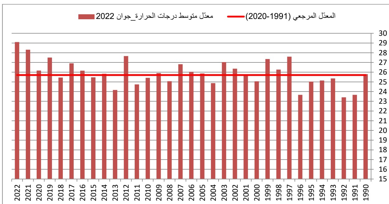
مقارنة معدل متوسط درجات الحرارة لشهر جوان بالمعدل المرجعي (1991-2020)
