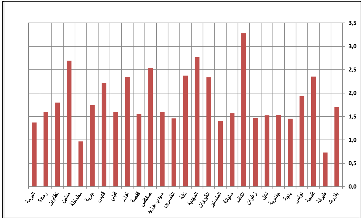
فارق معدل درجات الحرارة الصغرى لصيف 2022 عن المعدل المرجعي الموسمي (1991-2020)
