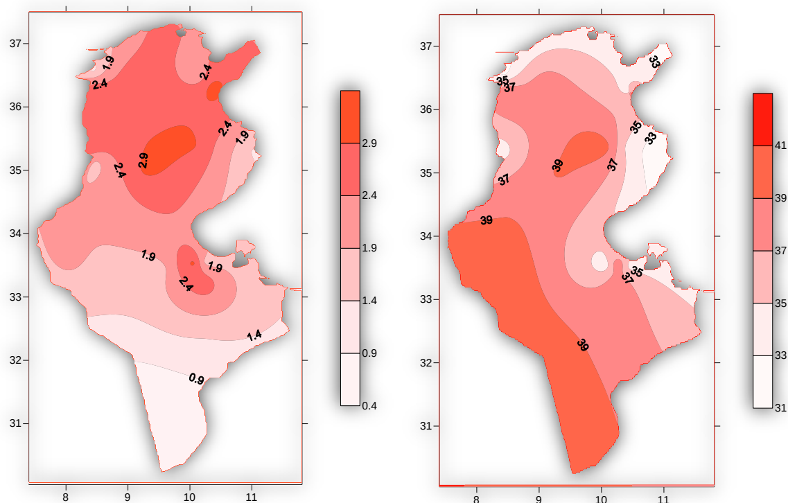
فارق معدلات الحرارة القصوى عن المعدلات المرجعية
