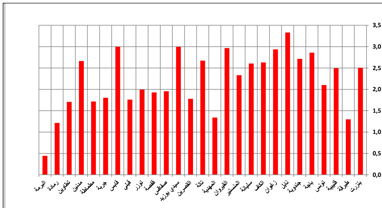
فارق معدلات الحرارة القصوى لصيف 2022 عن المعدل الموسمي المرجعي (2020-1991)
