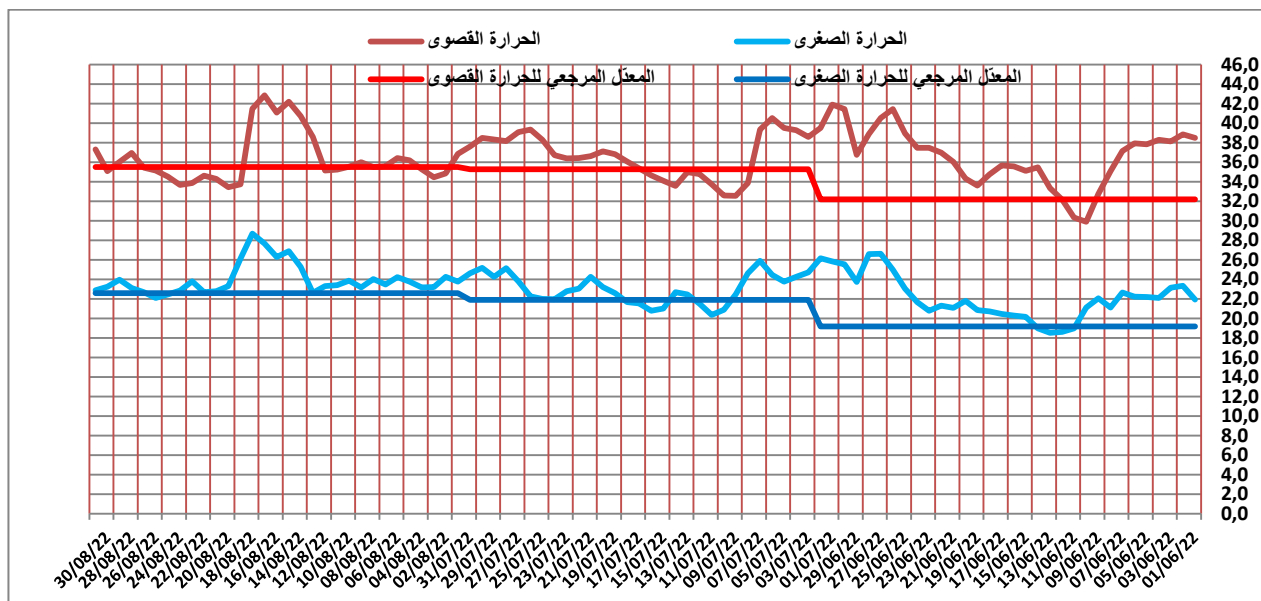
تطور درجات الحرارة الصغرى والقصوى اليومية خلال صيف 2022
