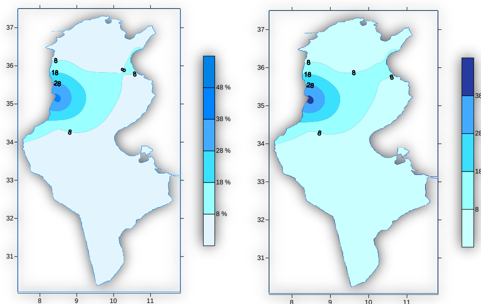
نسبة الأمطار الموسمية إلى المجموع المرجعي
