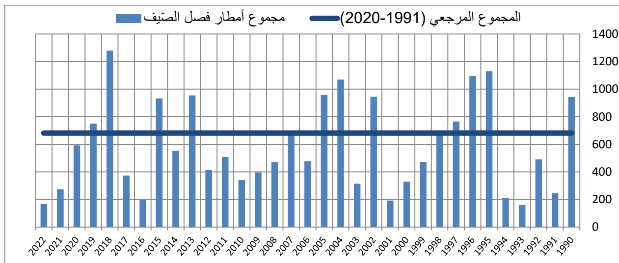
مقارنة مجموع الأمطار (27 محطة رئيسة) لصيف 2022 بالمجموع الموسمي المرجعي (1991-2020)
