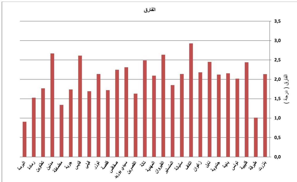
فارق معدل متوسط درجات الحرارة لصفيف 2022 عن المعدل المرجعي الموسمي (1991-2020)
