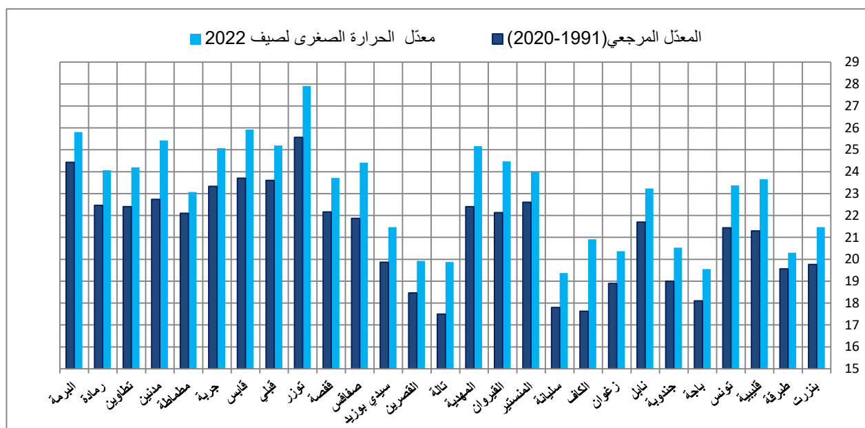
مقارنة معدل درجات الحرارة الصغرى لصيف 2022 بالمعدلات المرجعية الموسمية
