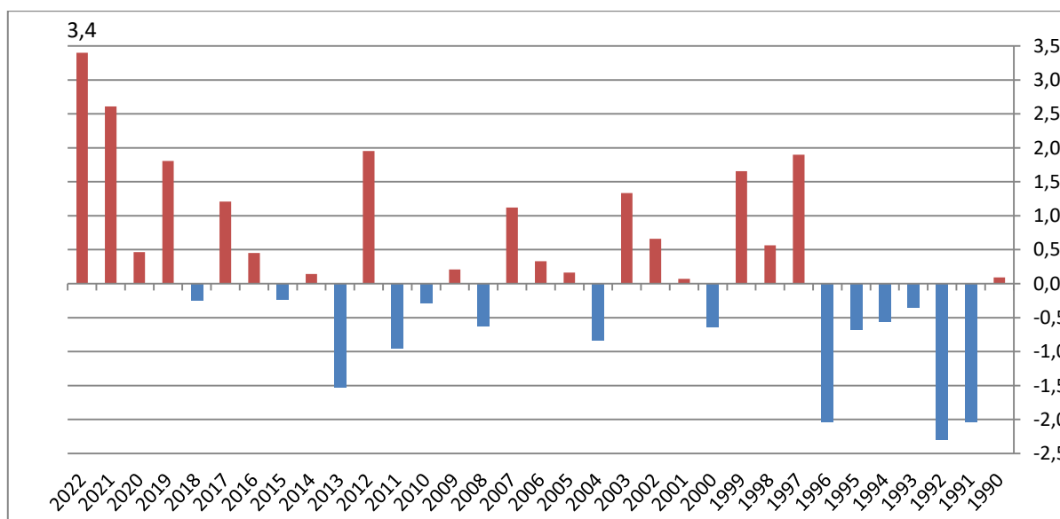
فارق معدّل متوسط درجات الحرارة لشهر جوان عن المعدل المرجعي (1991-2020)
