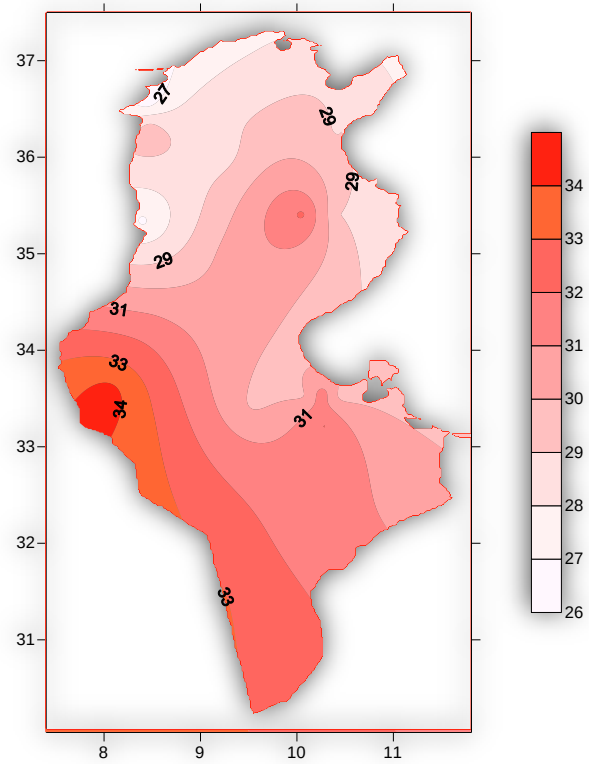
معدل متوسط درجات الحرارة (درجة)
