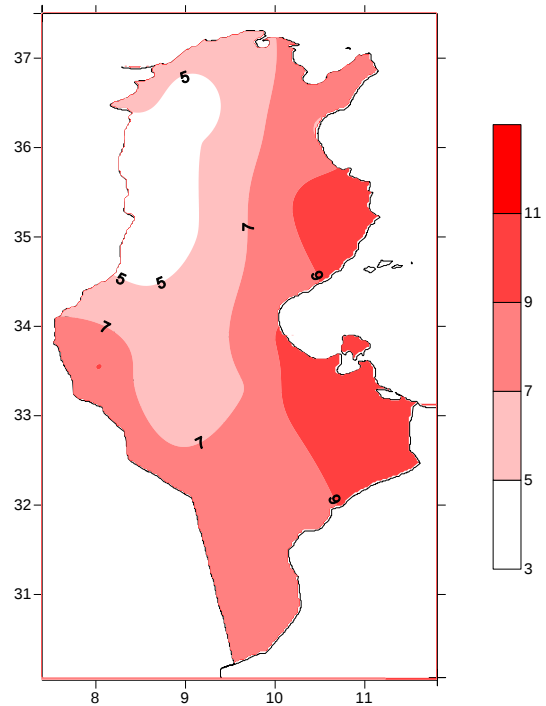
معدل درجات الحرارة الصغرى (درجة)
