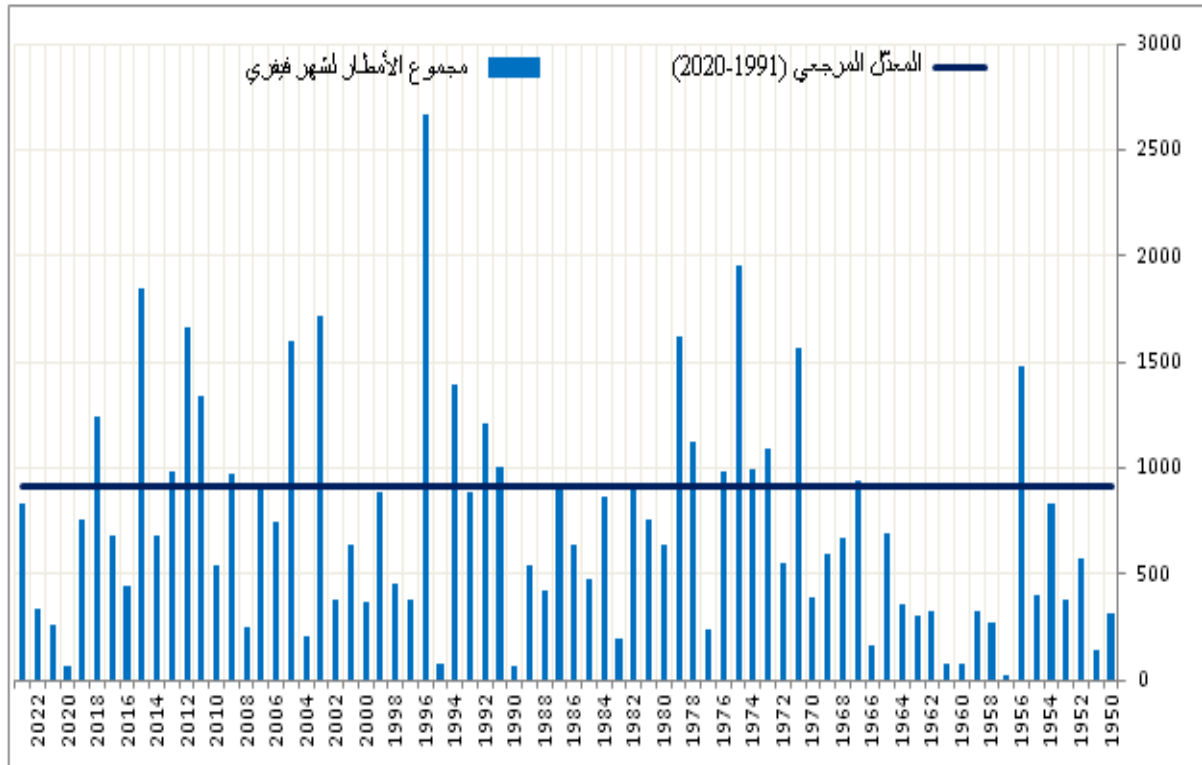
مجموع الأمطار الشهري بالبلاد التونسية خلال شهر فيفري منذ عام 1950
