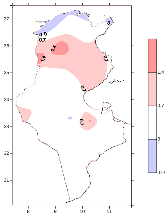
فارق متوسط درجات الحرارة عن المعدل المرجعي
