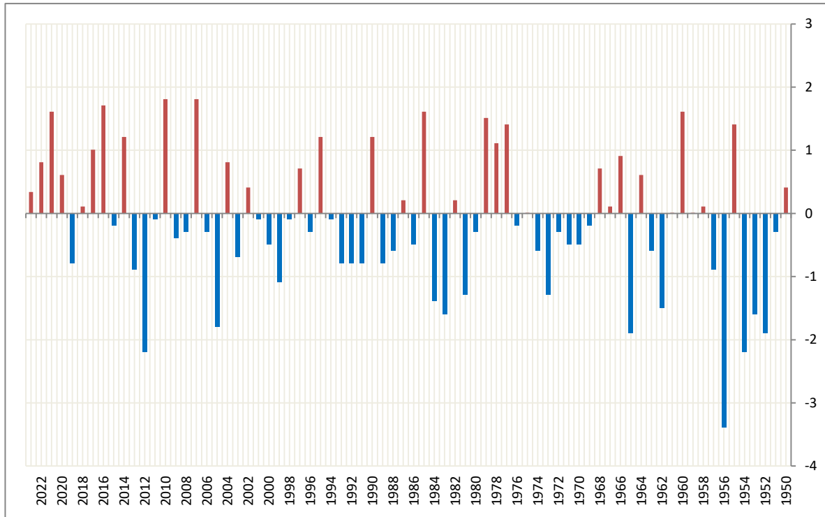
فارق درجات الحرارة الصغرى لشهر فيفري عن المعدلات المرجعية (2020-1991)
