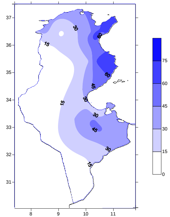
مجموع كميات الأمطار بالمحطات الرئيسية لشهر فيفري 2023 ( بالمليمتري )
