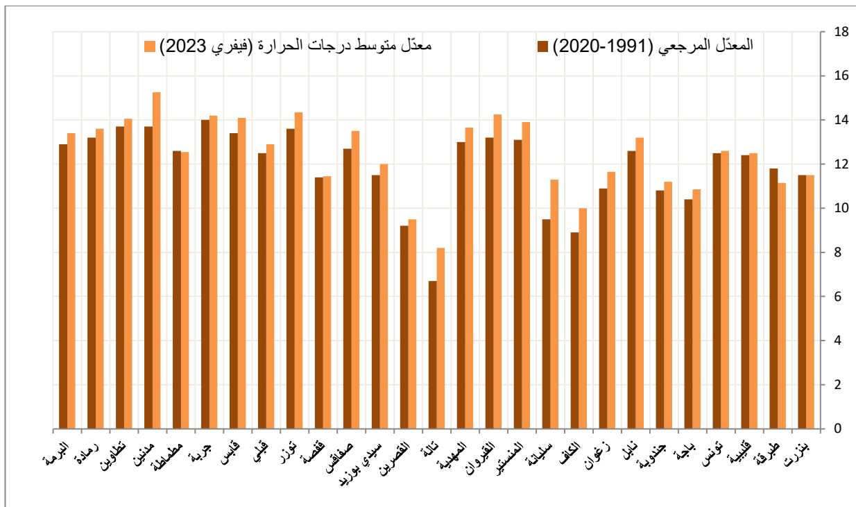
مقارنة متوسط درجات الحرارة لشهر فيفري 2023 بالمعدّلات المرجعية لشهر فيفري (1991-2020)
