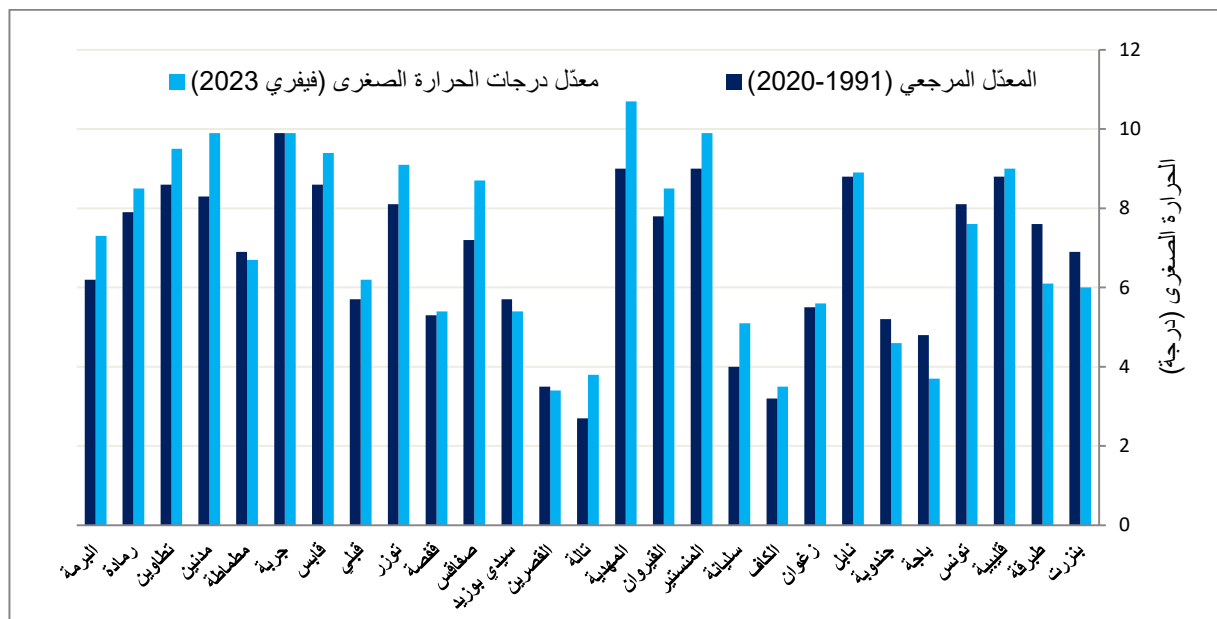
مقارنة معدل الحرارة الصغرى لشهر فيفري 2023 بالمعدّلات المرجعية (2020-1991)
