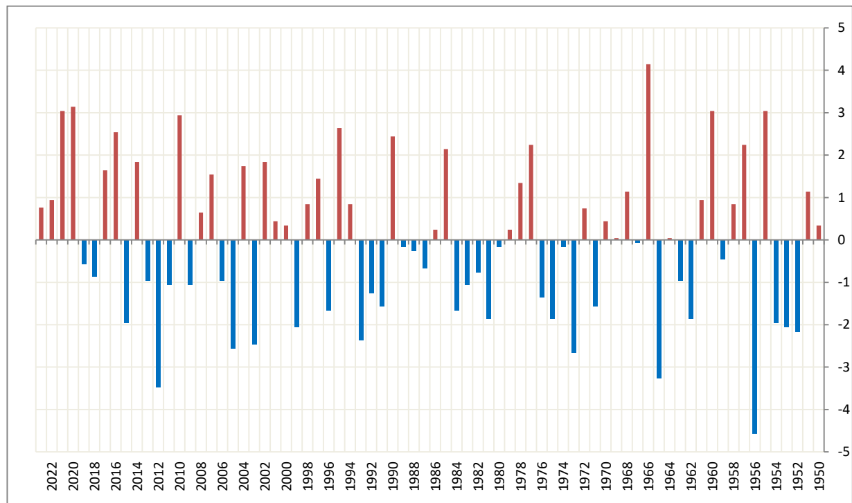
فارق درجات الحرارة القصوى لشهر فيفري عن المعدلات المرجعية (2020-1991)
