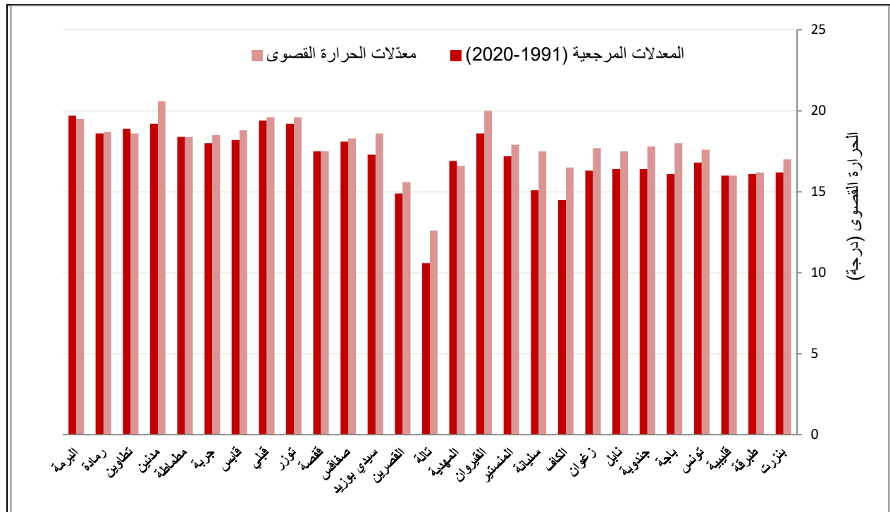
مقارنة معدل الحرارة القصوى لشهر فيفري 2023 بالمعدلات المرجعية (2020-1991)
