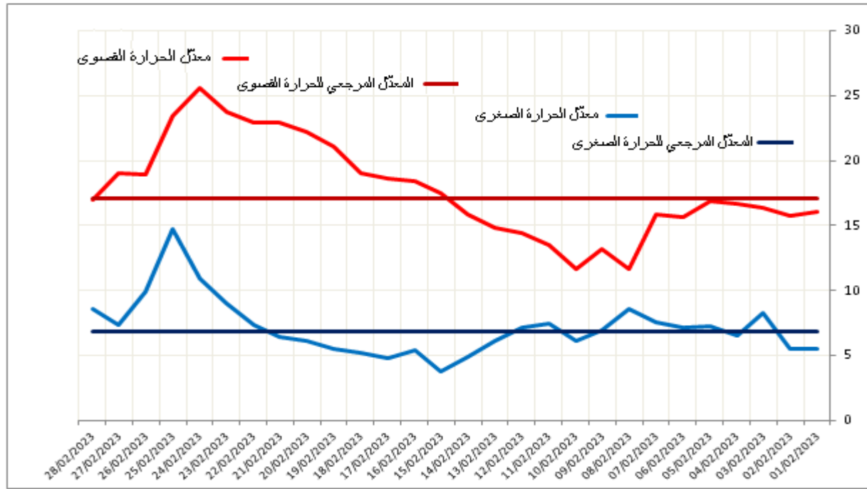
تطورات درجات الحرارة اليومية مقارنة بالمعدلات المرجعية لشهر فيفري
