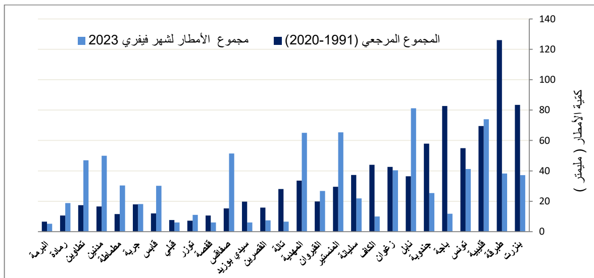
مقارنة مجموع الأمطار لشهر فيفري 2023 بالمعدّل المرجعي للشهر (2020-1991)
