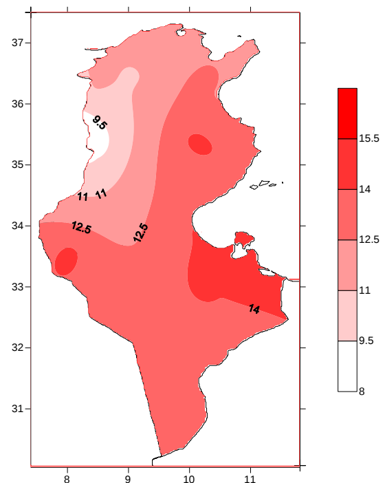
معدّل متوسط درجات الحرارة (درجة)
