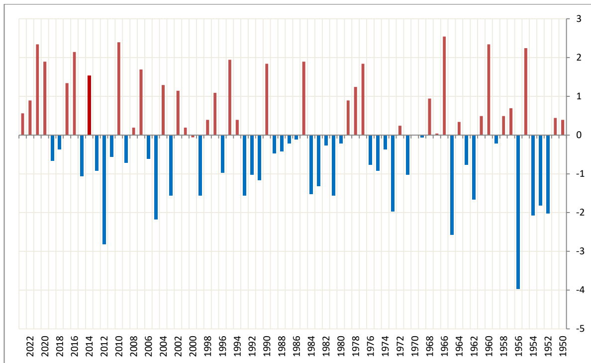
فارق معدّل متوسط درجات الحرارة لشهر فيفري عن المعدل المرجعي (1991-2020) منذ عام 1950
