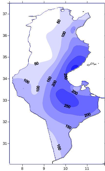
نسبة مجموع أمطار شهر فيفري 2023 إلى المعدل الشهري المرجعي ( % )
