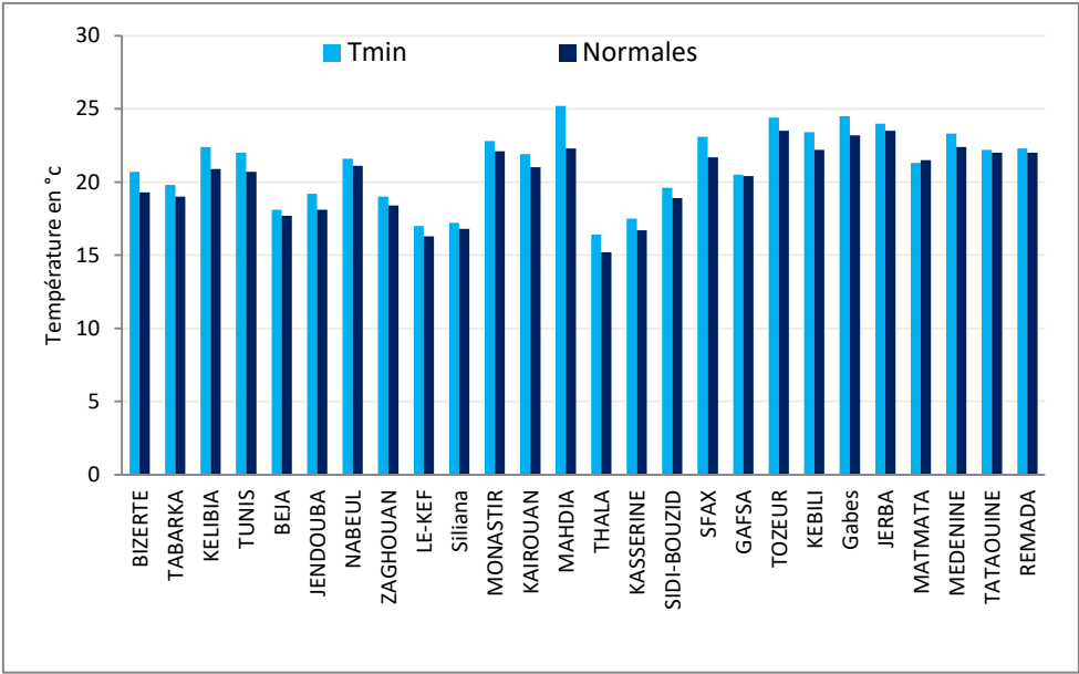
Comparaison des températures minimales aux normales du mois de Septembre 2025
