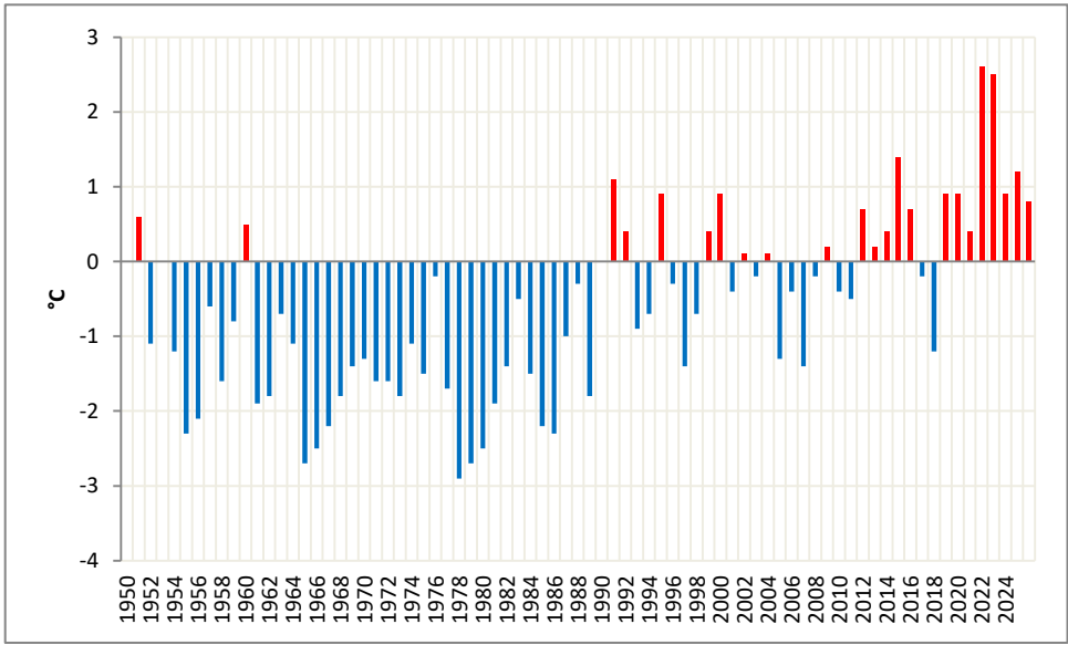
Ecarts à la normale (1991-2020) des températures minimales depuis 1950 : mois de Septembre
