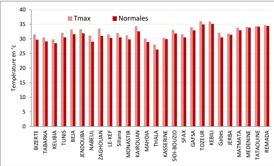
Comparaison des températures maximales aux normales du Mois de Septembre 2025
