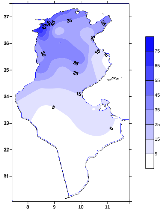
Cumul mensuel (mm) Septembre 2025
