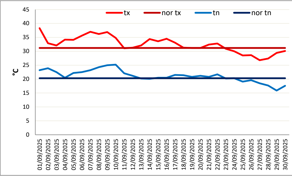
Evolutions des températures quotidiennes en Tunisie par rapport à la normale du mois de Septembre 2025
