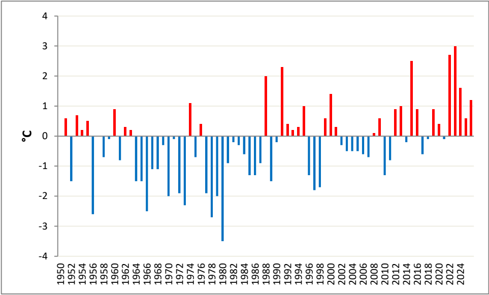
Ecart à la normale (1991-2020) des températures maximales depuis 1950 : mois de Septembre
