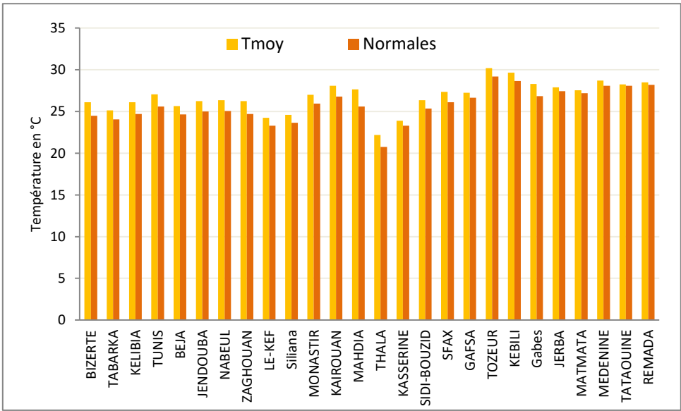
Comparaison des températures moyennes aux normales du mois de Septembre 2025
