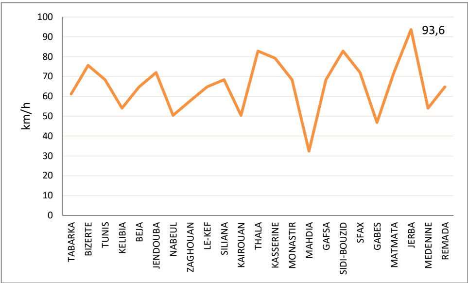
Vitesse maximale du vent (km/h) _ Septembre 2025
