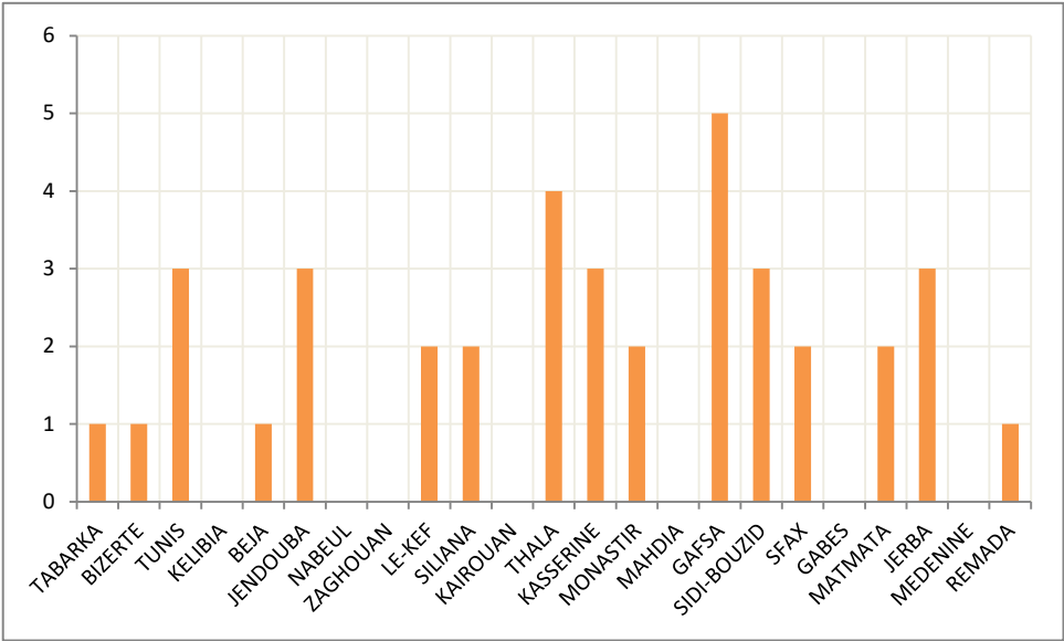
Nombres de jours avec vitesse du vent ≥ 60km/h Septembre 2025
